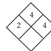
trinitrotoluene
