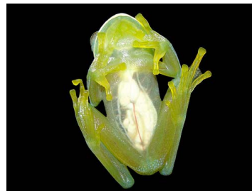
11 Vitreorana antisthenesi (FRR) CENTROLENIDAE
