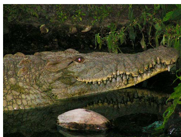
58 Crocodylus acutus (FRR) CROCODYLIDAE
