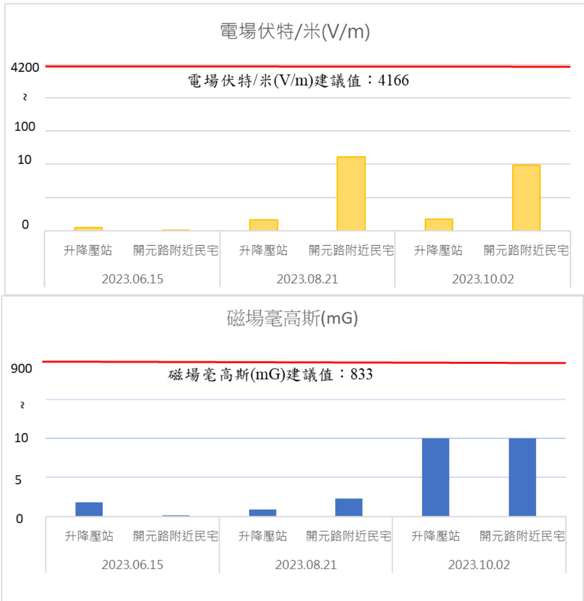
圖 3.1.12-1 歷季電磁場量測結果示意圖
