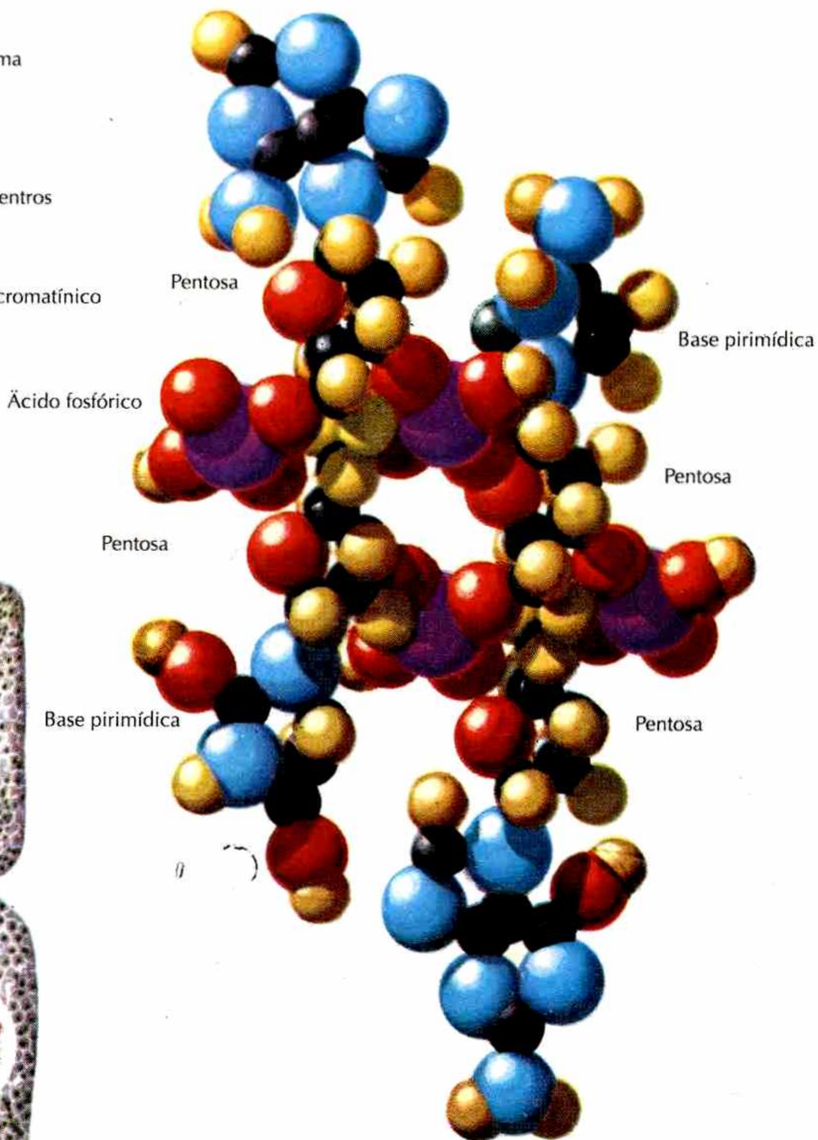
Fig. 2.- Molécula de ácido timonucleínico de 4 nucleótidos.
