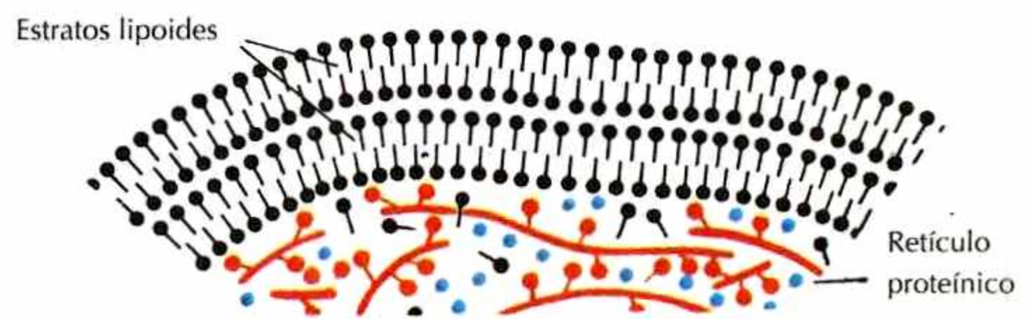
Fig. 5.- Esquema de la estructura molecular de la membrana protoplasmática.
