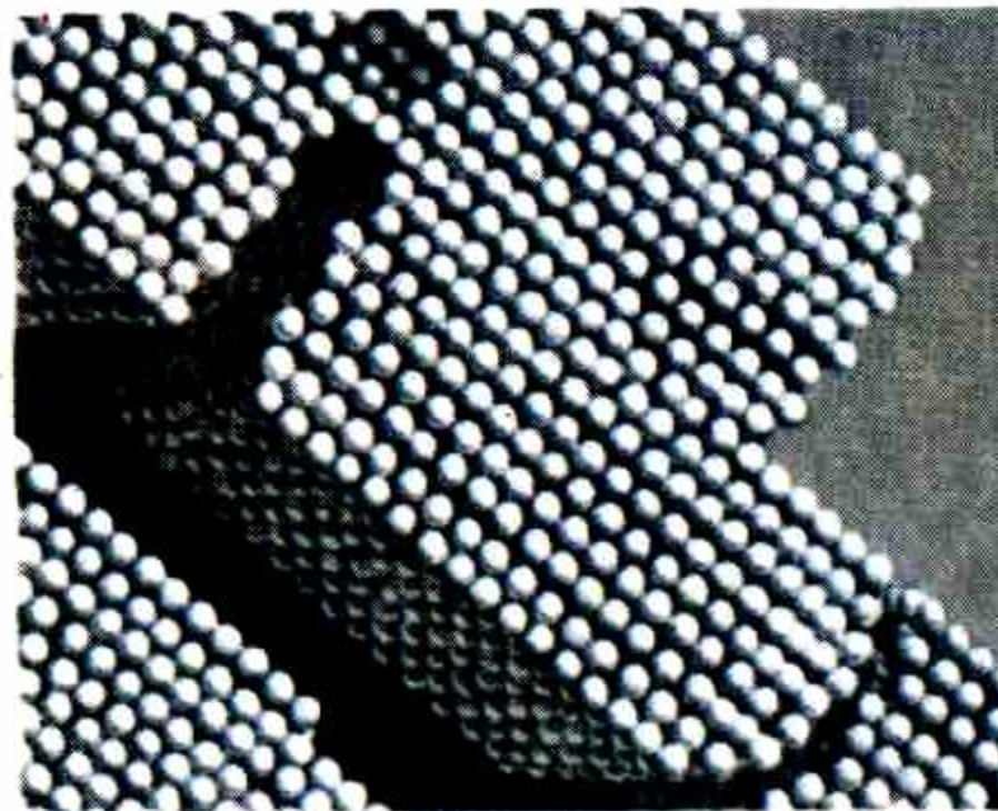
Fig. 8.- virus causante del "mosaico de la judía" completamente cristalizado. Aumento de 60.000 diámetros.
