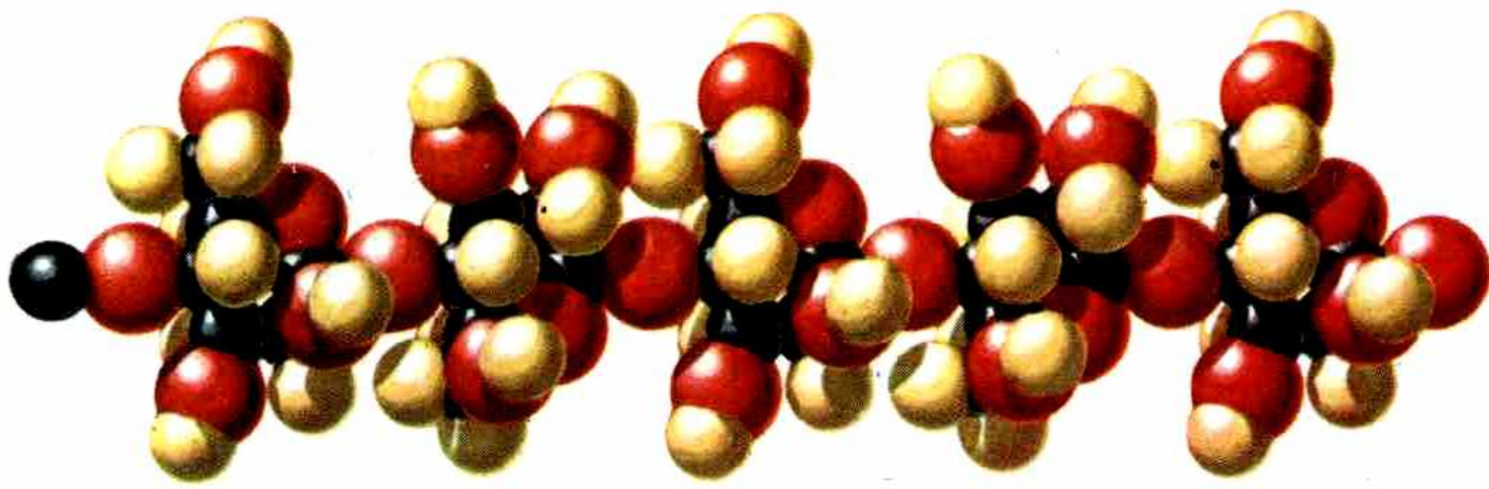
Fig. 1.- Fragmento de una molécula de celulosa.
