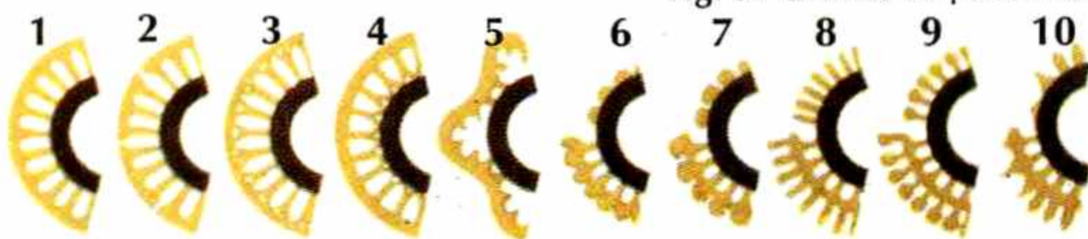
Fig. 4.- Esquema estructural del grano de polen. La endexina, en oscuro, y la ectexina, en claro.
