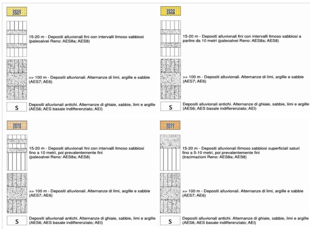
Figura 8.2 – Schemi dei rapporti stratigrafici rappresentativi delle zone di attenzione per instabilità
