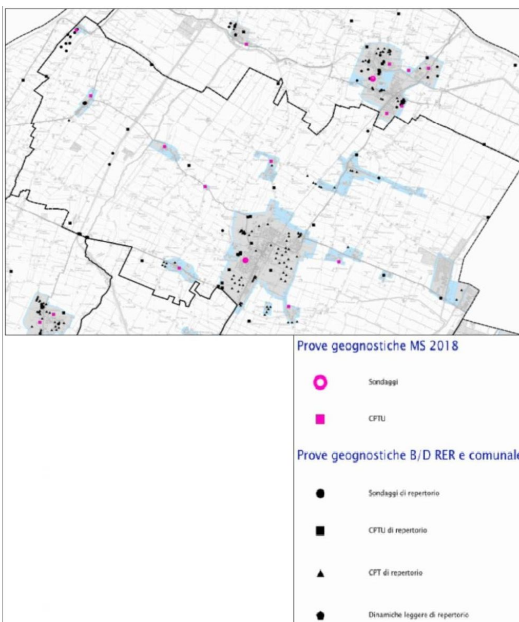
Figura 4.1- Localizzazione delle indagini geognostiche (di repertorio e di nuova esecuzione) disponibili per lo studio di microzonazione sismica
