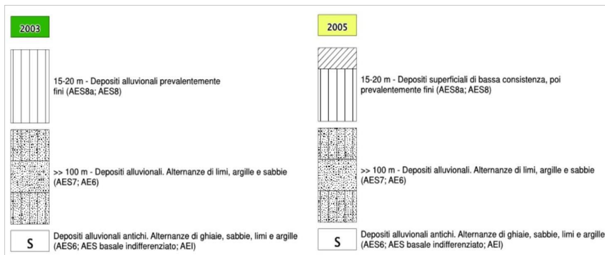
Figura 8.1 – Schemi dei rapporti stratigrafici rappresentativi delle zone stabili
