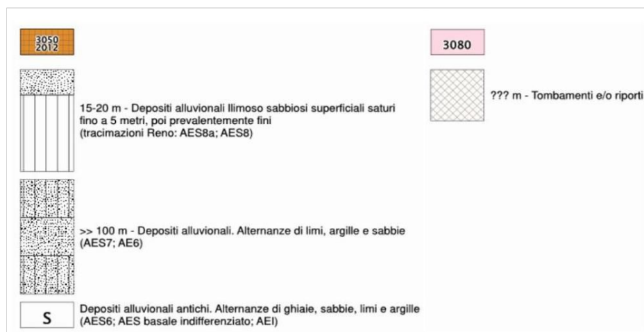
Figura 8.3 – Schemi dei rapporti stratigrafici rappresentativi delle zone di attenzione per instabilità
