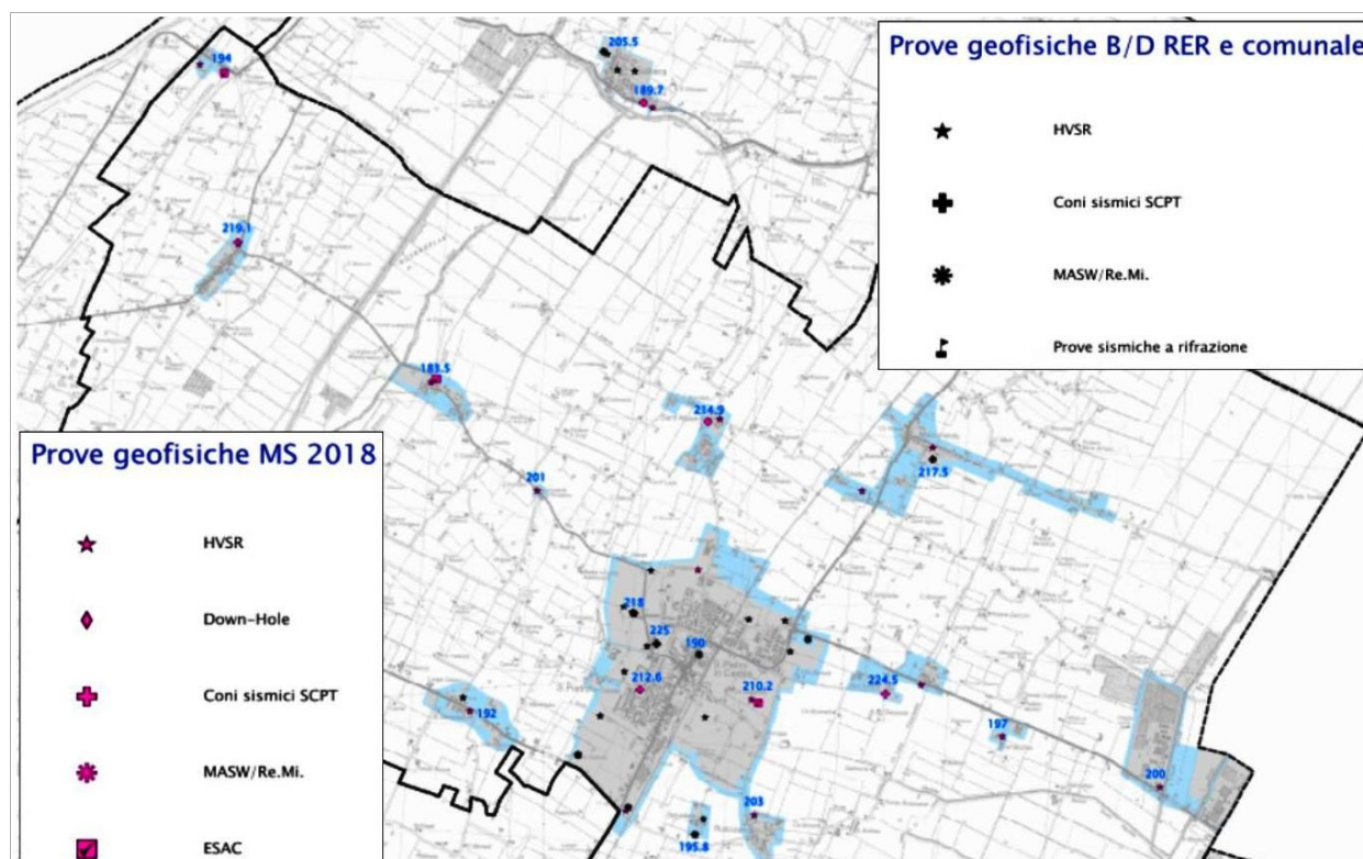
Figura 5.8 – Indagini geofisiche disponibili nel territorio di San Pietro in Casale con calcolo della V_{s30} . È indicata anche la tipologia di prova
