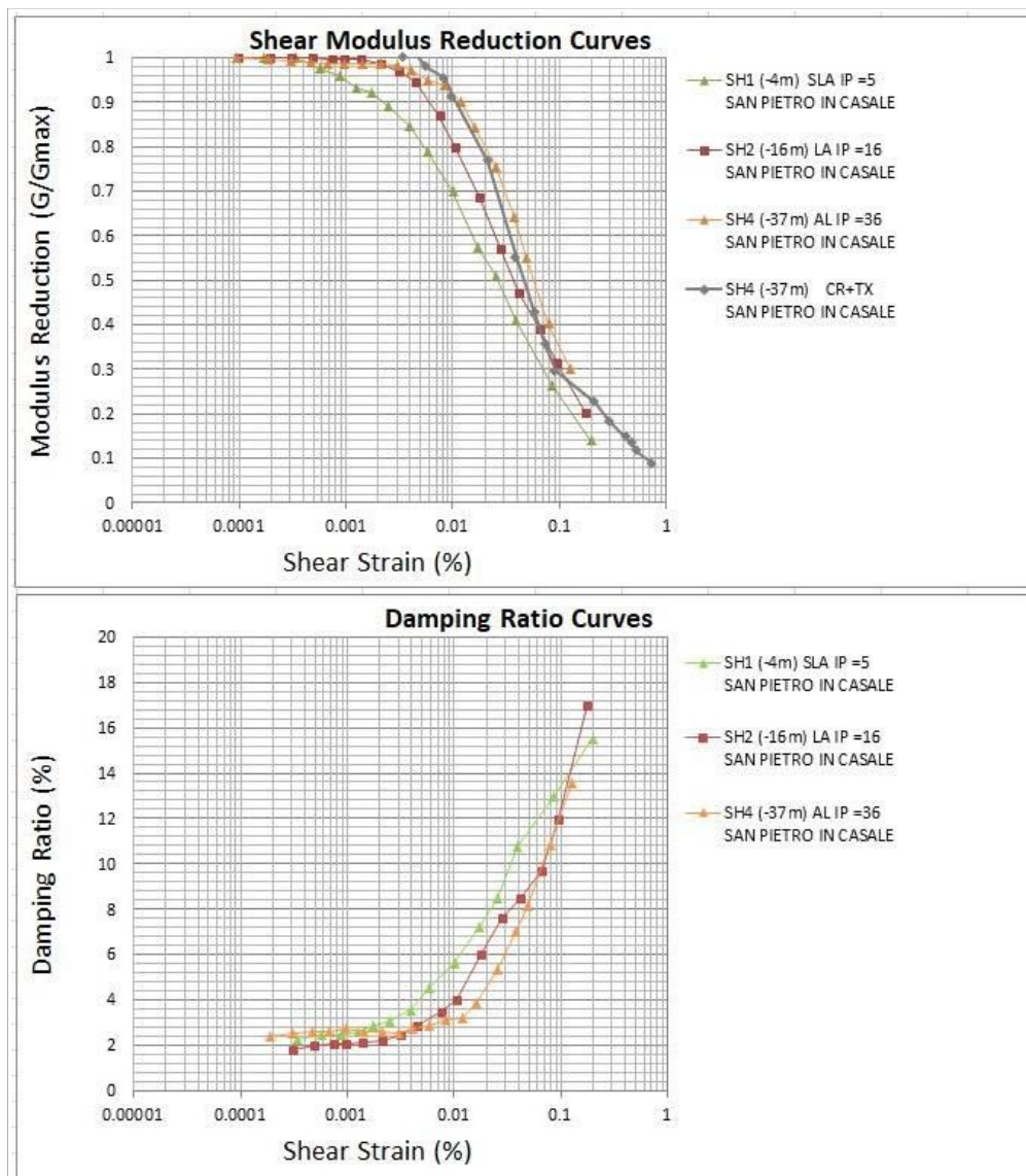
Figura 5.2 - Curve di decadimento dei sedimenti fini di San Pietro in Casale (sondaggio eseguito nel Capoluogo)
