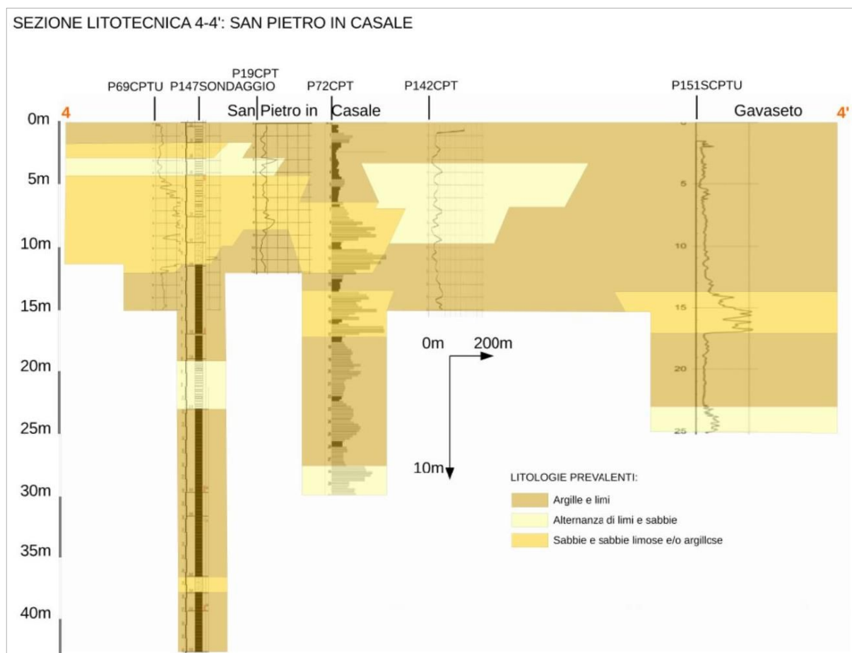
Figura 5.5- Sezione litotecnica 4-4' (Capoluogo) elaborata per questo studio
