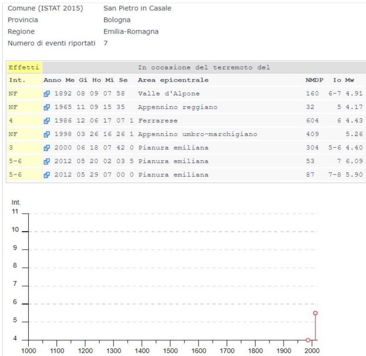
Figura 2.1 - Elenco e diagramma cronologico (con macrointensità stimate) degli eventi sismici significativi per il Comune di San Pietro in Casale (fonte: INGV - Database Macrosismico Italiano 2015)
