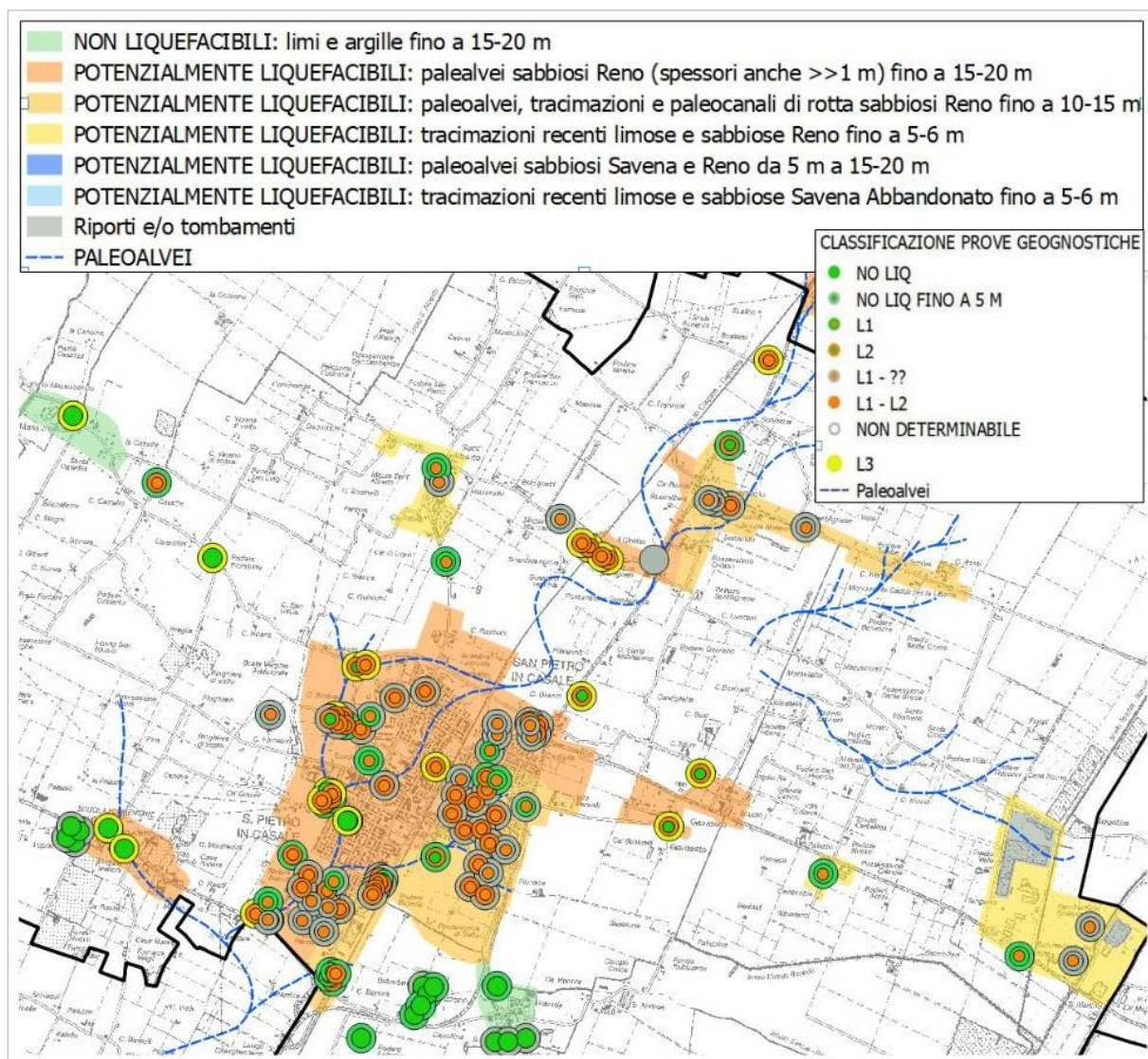
Figura 6.3 - Classificazione dei punti di controllo geognostici finalizzata alla ricostruzione delle zone di potenziale liquefabilità in base alla presenza di strati granulari in falda
