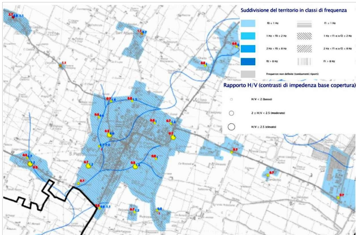
Figura 5.9 - Suddivisione del territorio urbano/urbanizzabile di San Pietro in Casale in classi di frequenza naturale dei terreni. I colori rappresentano classi differenti. L'ampiezza dei cerchi classifica le massime amplificazioni spettrali ricavate dalle registrazioni HVSR
