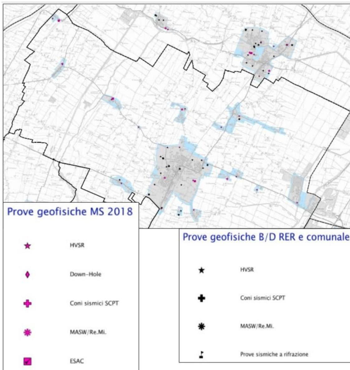
Figura 4.2- Localizzazione delle indagini geofisiche (di repertorio e di nuova esecuzione) disponibili per lo studio di microzonazione sismica
