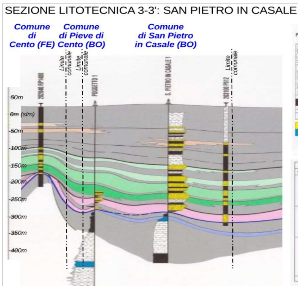
Figura 5.3 – Sezioni litotecniche di riferimento per lo studio di MS (Unione Reno Galliera e dettaglio di S. P. in Casale)
