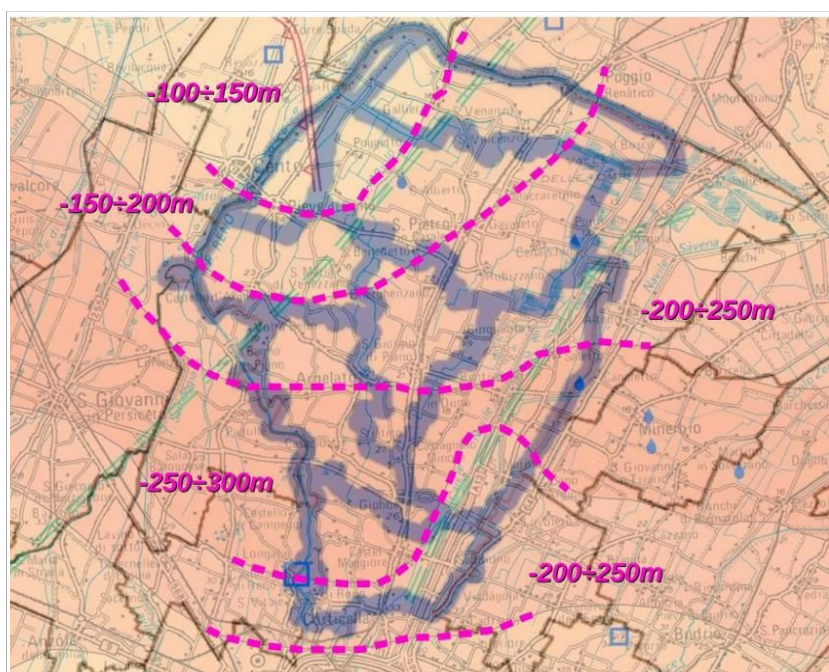
Figura 5.6 - Stralcio della Carta Sismotettonica della Regione Emilia-Romagna ed aree limitrofe (RER, 2016). Sono sovrapposti i confini comunali dei Comuni dell'Unione e rimarcate le isobate della base del Sintema AES (m slm)
