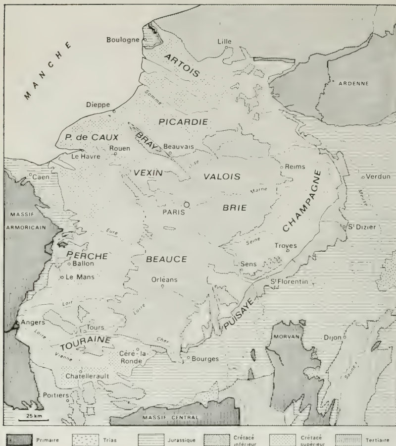
CARTE GEOLOGIQUE SCHEMATIQUE DU BASSIN DE PARIS
