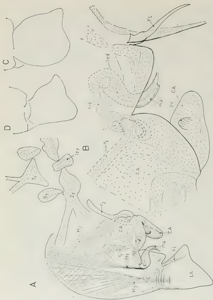
Text-fig. 7. Organe copulateur, mâle. A, B, E, n. sp. A ( Gran Piedra ). A, vue générale de la partie droite, face dorsale (ou interne); B, détail, de la face ventrale (ou externe). C-D, E. bromeliarium F. Müll. le lobe A. C, d'après F. Müller, 1881. D, d'après Pinto et Purper, 1790 (LA — le lobe A; M1 — M3 — muscles érecteurs intrapénien. CA, crochet accessoire; I, r2 — rainures sclérisées supportant les insertions musculaires; ma — manchon; O — orifice proximal du tube éjaculateur; tep — tube éjaculateur, région proximale; ted — tube éjaculateur, région distale; Fl — flagelle; Pr — protubérance; Izy — interzygum; Zy — zygum; st — sternyx; tro — trophis; Fu — lobe furcal).
