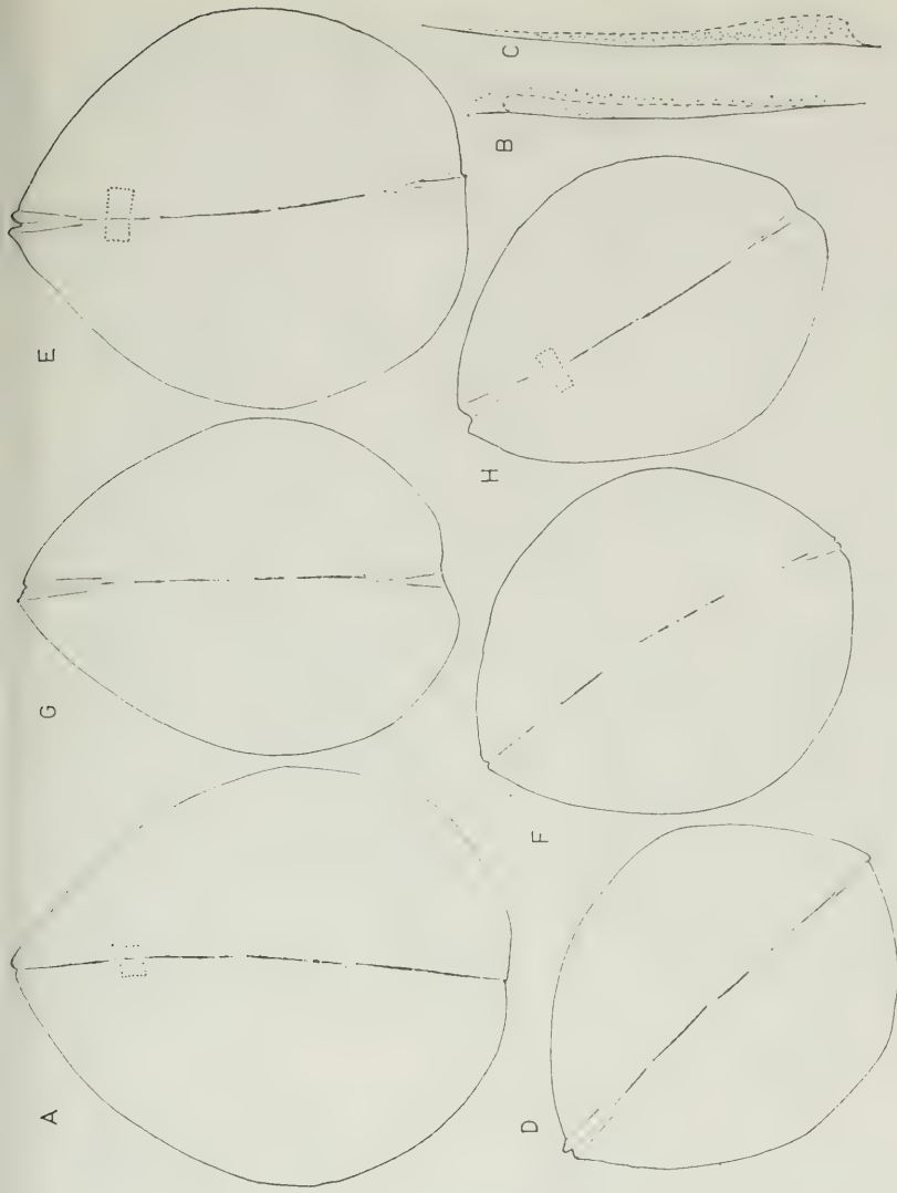
Text-fig. 5. Coquilles d' Elpidium en vue dorsale. A-D, E., n. sp. C. A, femelle. B, C, fosses antérieure et postérieure de la charnière de la valve droite femelle. D, mâle. E, F-E., n. sp. B, E, femelle. F, mâle. G, H, E., n. sp. A (exemplaires de Rio Indio). G, femelle. H, mâle. (Dimensions in text.)
