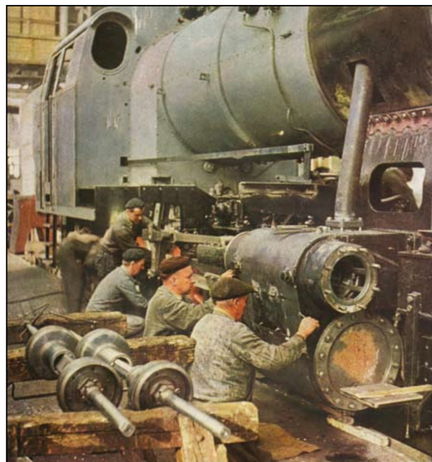
Montáž lokomotivy
