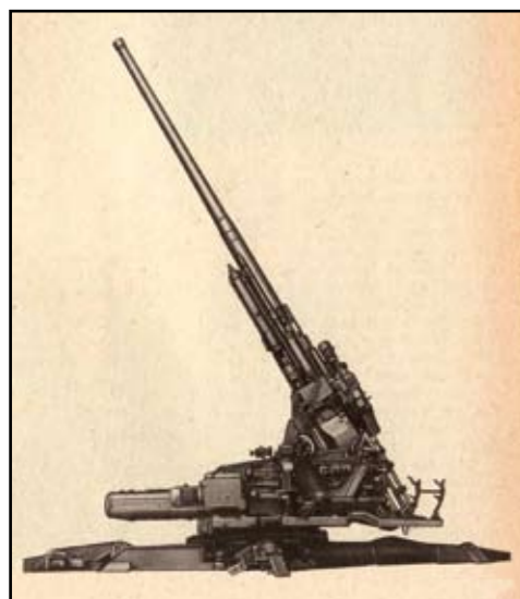
130mm protiletadlový kanón KS-30
