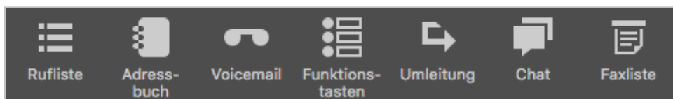
Abbildung 31 - Element „Menü-Icons“
