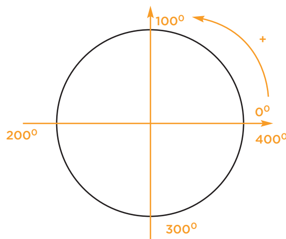
Figura 10. Medida de ángulos con graduación centesimal en sentido antihorario
