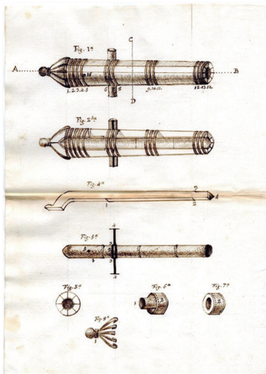
Dibujo del proyecto para hacer cañones de hierro forjado, sustituyendo los de hierro común. 1809. AGMS.
