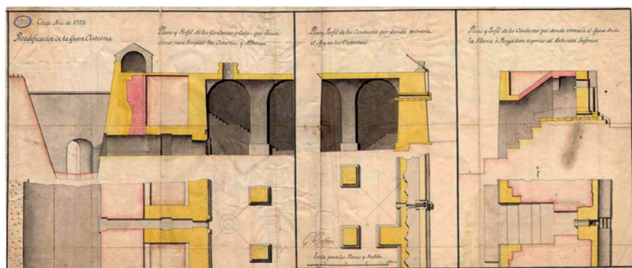
Plano y perfil para la reedificación de la Gran Cisterna. 1723. Archivo Intermedio Militar de Ceuta.
