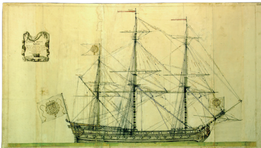
Perfil y jarcia de un navío español. Álbum de construcción naval del marqués de la Victoria (1719-1756). Hoja 125. Archivo del Museo Naval.
