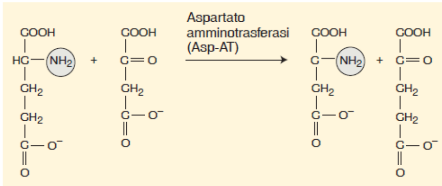
Glutammato Ossalacetato
