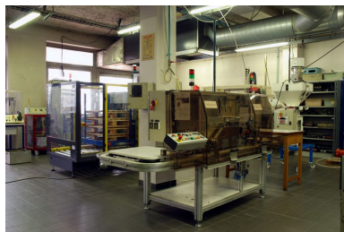
Machine à conteneuriser des cachets dans des flacons Phot. Catherine Guégan IVR82_20116901933NUCA
