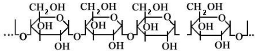
Figura I. 3. Amilosa.
