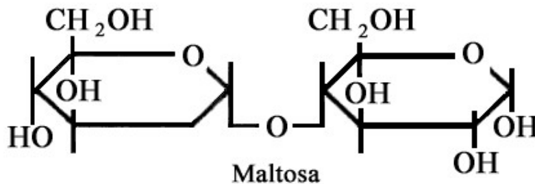
Figura I. 2. Maltosa
