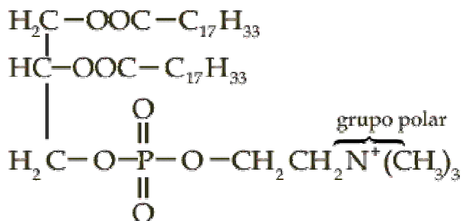
Figura III. 3. Leticina típica.
