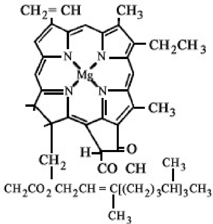
Figura III. 5. Clorofila a.
