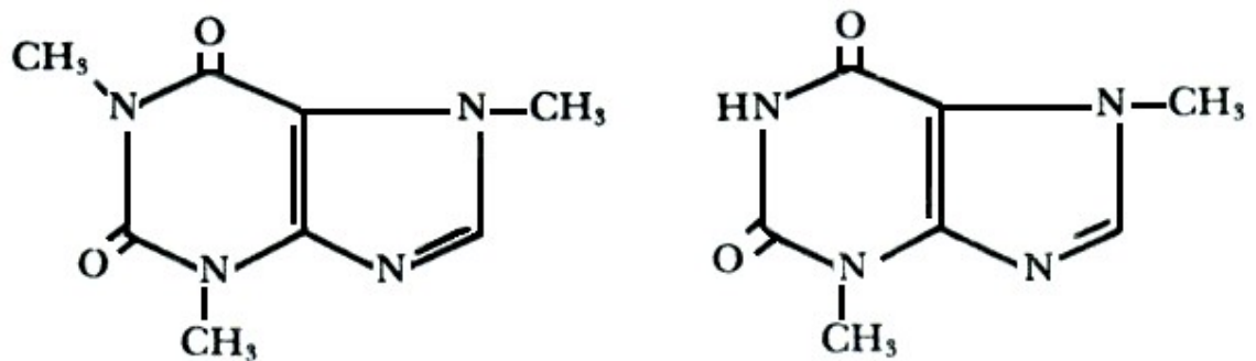
Figura IV. 1. Cafeína. Teobromina.
