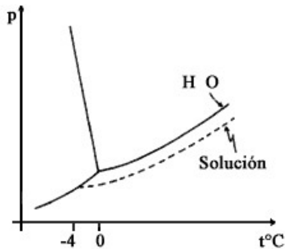
Temperatura de congelación de una solución
