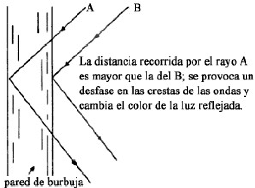
Figura V. 4. Fenómeno de interferencia.
