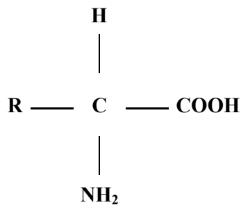
Figura I.5. Aminoácido
