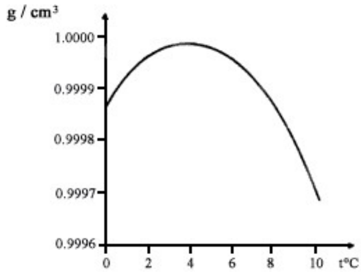
Densidad del H 2 O de 0 a 10°C
