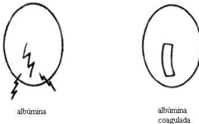
Figura II. 9. Acción de sal en la albúmina.
