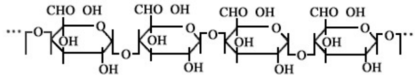
Figura I. 4. Celulosa.
