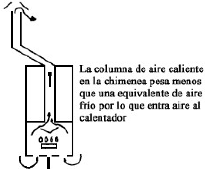
Figura II. 1. Chimenea de calentador doméstico.
