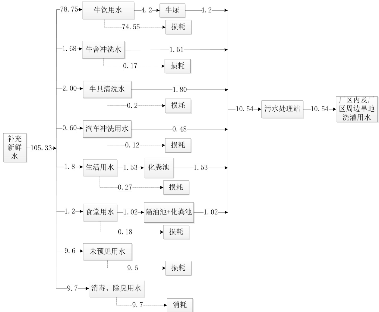
图 2.1-1 本项目水平衡图 (m 3 /d)
