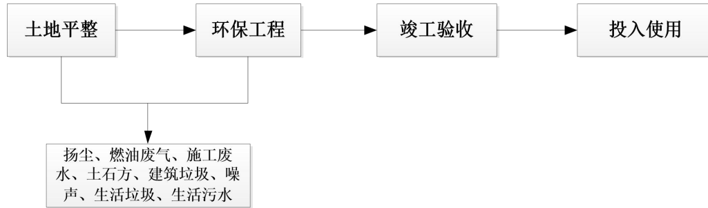
图 2.2-1 施工工艺流程图及产污节点图
