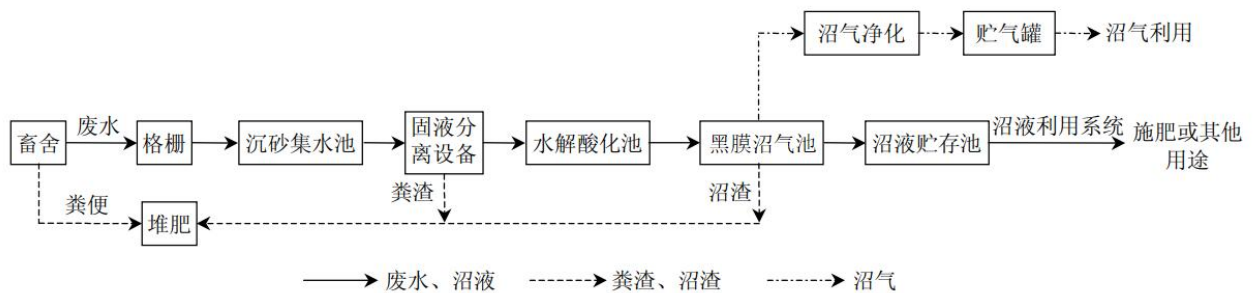
图 2.2-4 污水处理站处理工艺流程图
