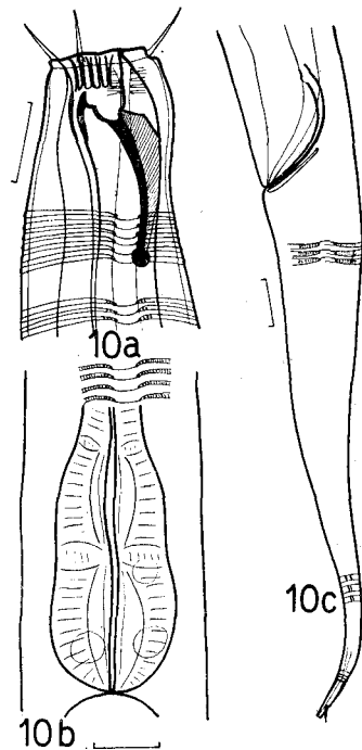
Fig. 10. Spilophorella tollenifera n. sp. a, Anterior end of male; b, pharyngeal bulb; c, posterior end of male.
