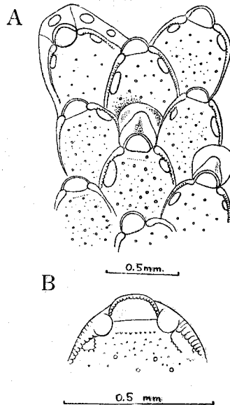
Fig. 9. Micropora coriacea (Johnston)
