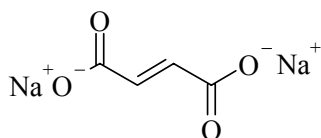
di-sodium fumarate
