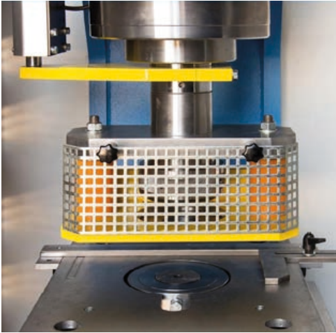
Optional punch tooling-set Optionales Stanzwerkzeugsatz Jeu d'outils de poinçonnage en option Juego de punzones opcional
