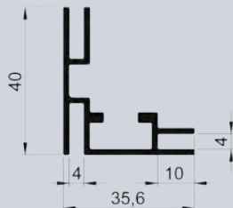
FSB41TX-CL
