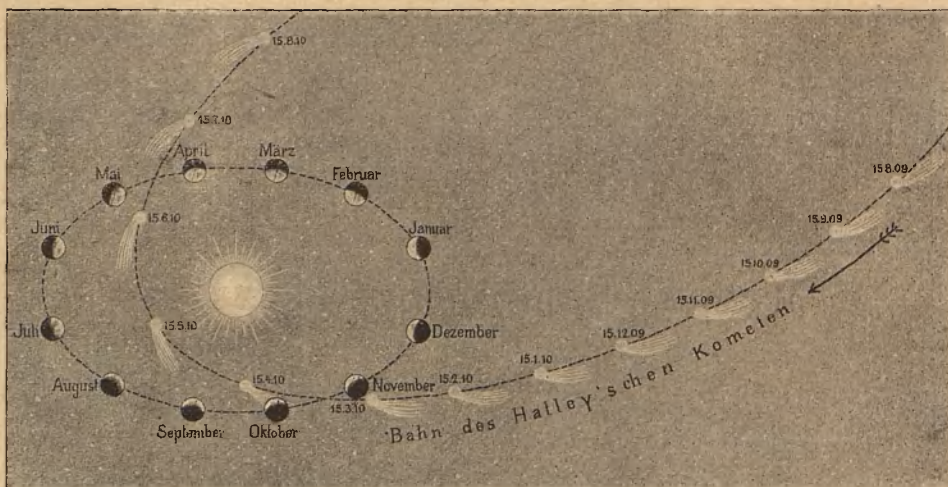
Die Bahn des Halley'schen Kometen und der Erde.
