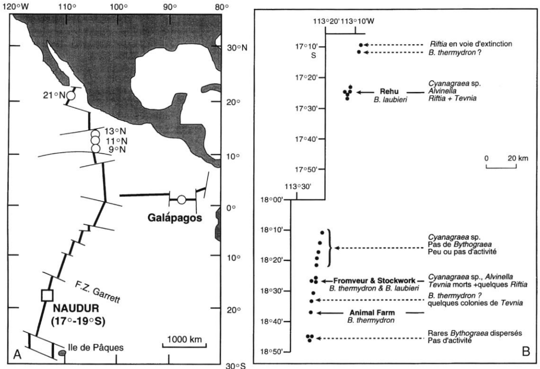
FIG. 1. — A, carte de la dorsale du Pacifique oriental indiquant la position des sites hydrothermaux connus du Pacifique oriental et de la zone explorée par la mission Naudur ; B, localisation des plongées de la mission Naudur ; à gauche sont indiqués, par des points noirs, les sites sur lesquels les crabes ont été récoltés ; la colonne de droite signale la présence des crabes identifiés à partir des observations vidéoscopiques, ainsi que celle des vestimentifères et des polychètes.
