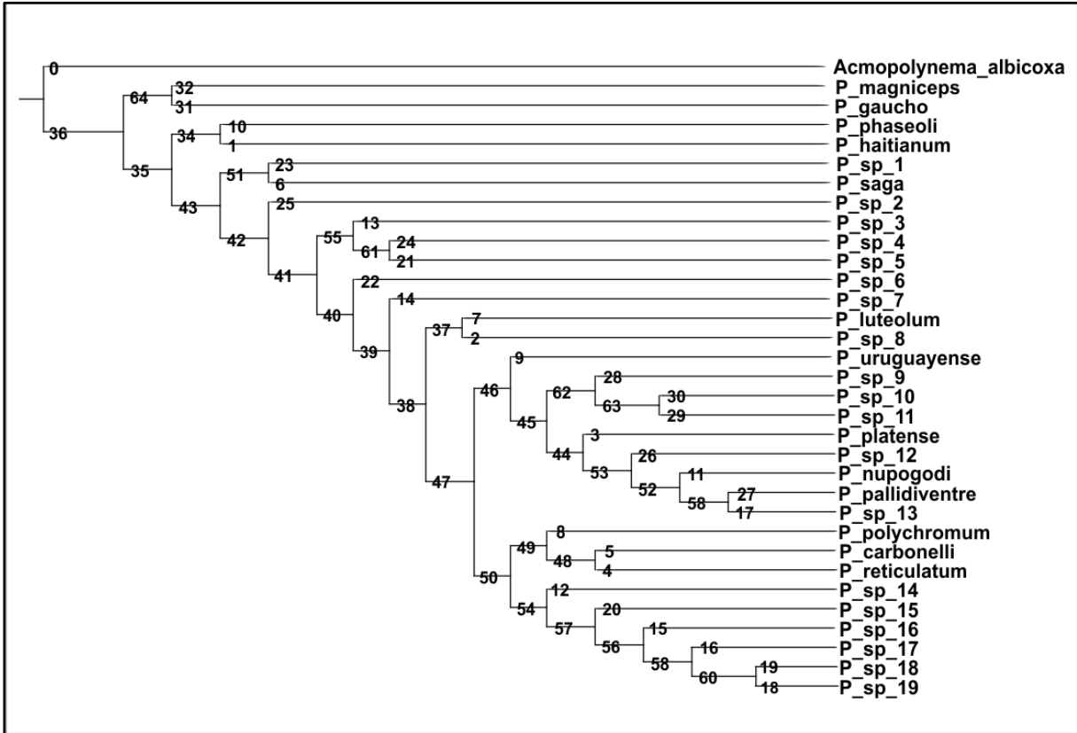
Fig. 50: Cladograma más parsimonioso.
