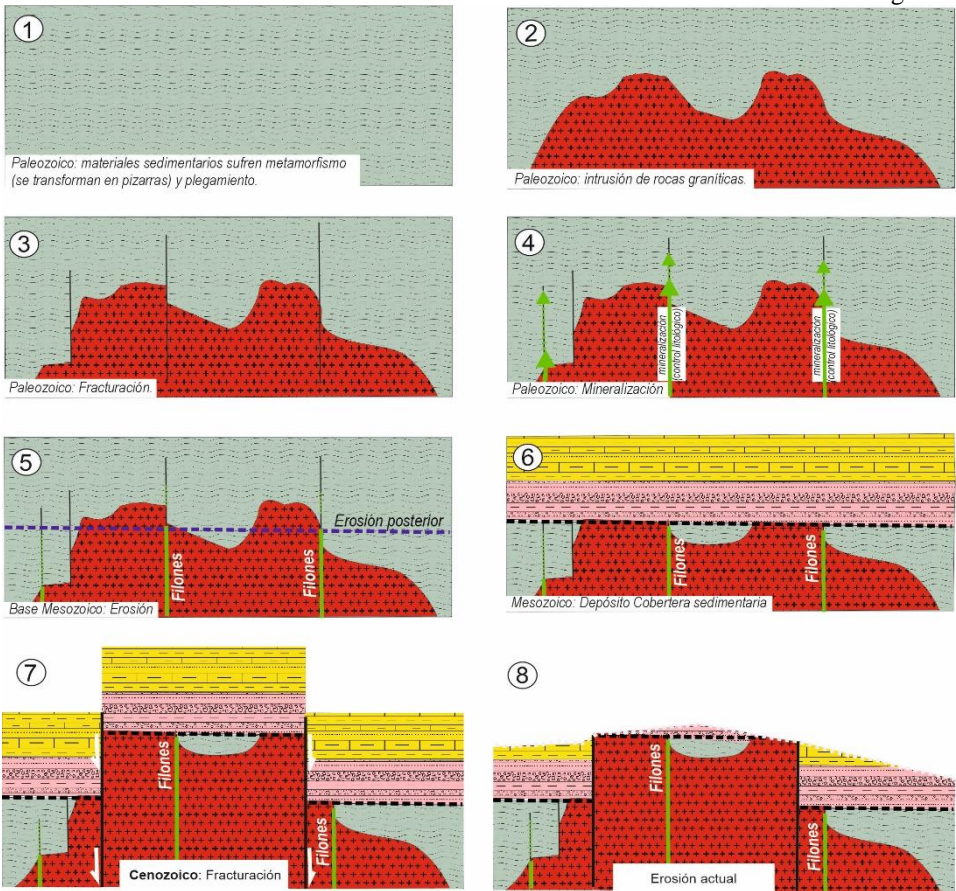
Fig. 2: Esquemas que representan la historia geológica del sector.
