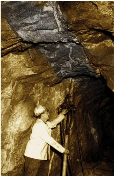
Fig. 3: Filón de galena en una antigua galería del distrito minero (fondo histórico).
