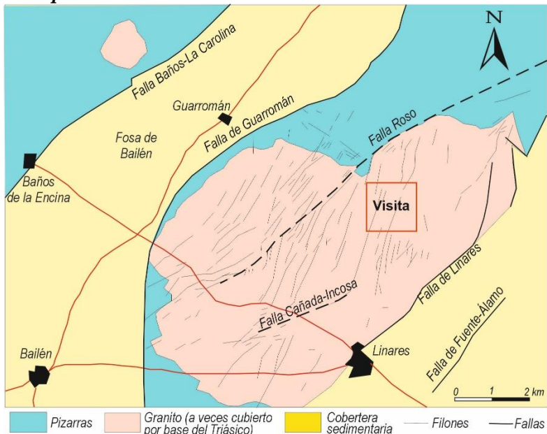
Fig. 1: Cartografía geológica regional simplificada.
