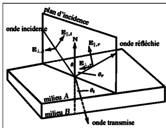
Fig. 4.6. Définition des composants du vecteur électrique [MIGNOT, 2004-2005].
