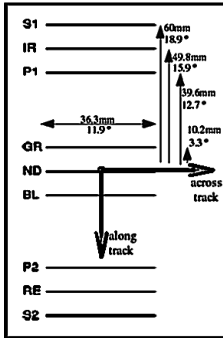
3.10.b Position physique sur le plan focal
