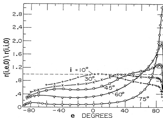
Fig. 5.10. Le pic de spécularité a lieu parfois à des angles d'émergence plus élevés.
