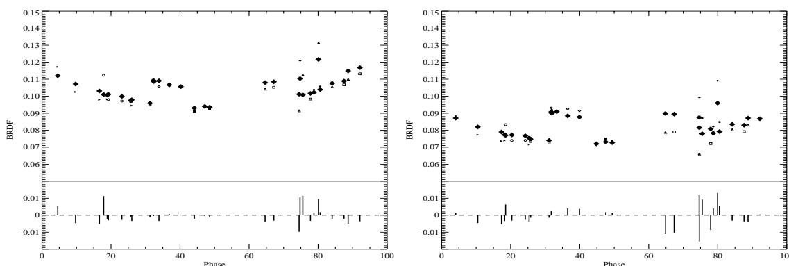
3.5.a Point "Red" 3.5.b Point "Green" Fig. 3.5. Fonction de phase modélisée et mesurée; étude des résidus en fonction de la phase. Les losanges désignent les réflectances modélisées, les barres verticales : les résidus (mesures-modèles).
