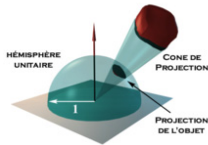
Fig. 2. Représentation d'un angle solide [Claustres, 1999-2000]
