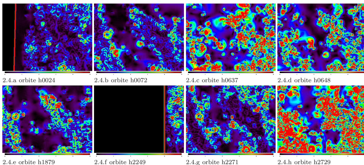
Fig. 2.4. Pentés obtenues au centre de Gusev à partir des MNT de chaque orbite HRSC. (Résolution : "100m" ; Champ : 80*40km) Les remparts du cratère Thyra apparaissent en haut à droite. L'échelle de couleurs s'étend de 0 à 10°. La couverture spatiale est identique à la figure Fig. 2.5 .
