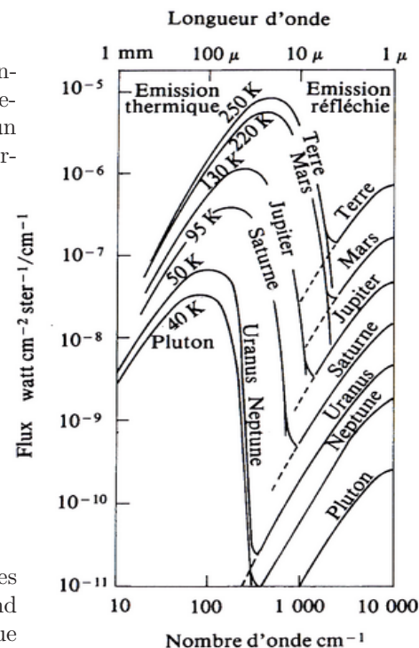
Fig. 4.5. Spectres thermiques et réfléchis des planètes
