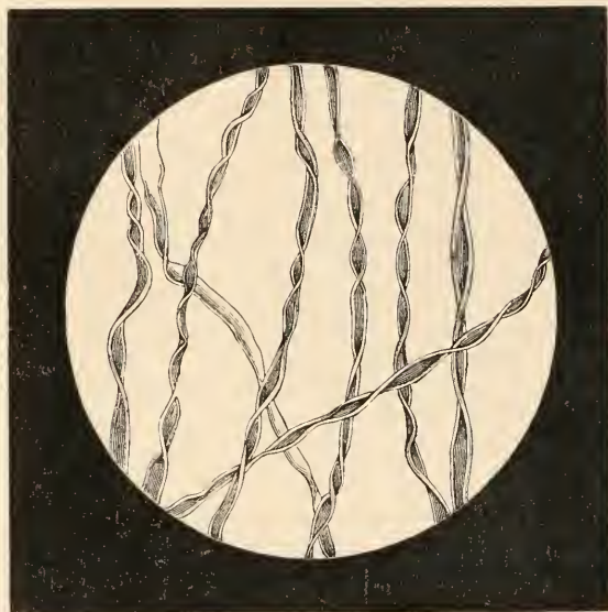
Fig. 5.—Fibres of American Cotton. × 225.
