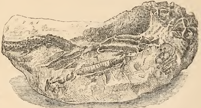
Fig. 47.— Meyeria Vectensis , McCoy.
