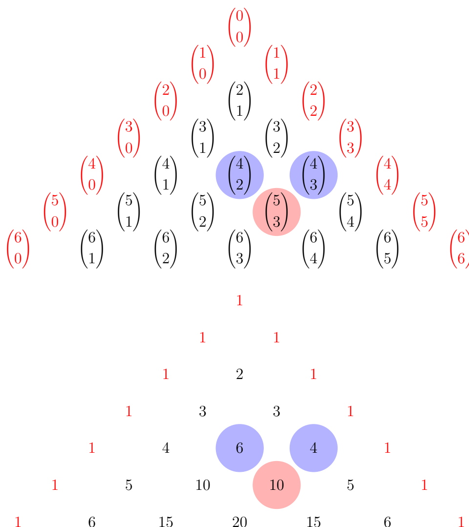
Obrázek 1.7: Pascalův trojúhelník.
