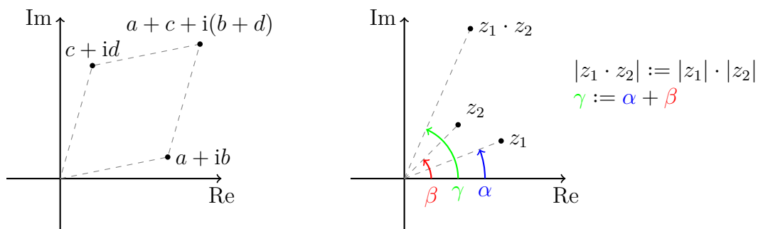
Obrázek 1.5: Geometrická interpretace operace sčítání a násobení komplexních čísel.
