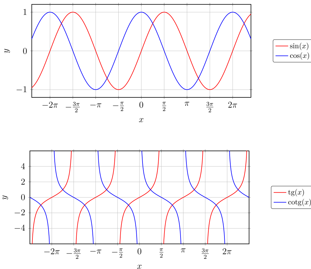
Obrázek 3.5: Trigonometrické funkce \sin , \cos , \operatorname{tg} a \operatorname{ctg} .
