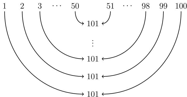
Obrázek 1.6: Gaussův trik.
