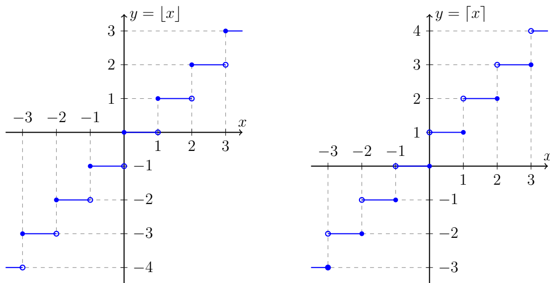
Obrázek 3.8: Grafy dolní (vlevo) a horní (vpravo) celé části.
