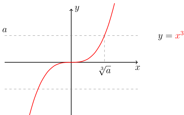
Obrázek 3.6: Konstrukce liché odmocniny čísla a .
