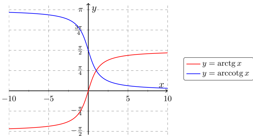
Obrázek 3.13: Grafy funkcí \arctg x a \arccotg x .
