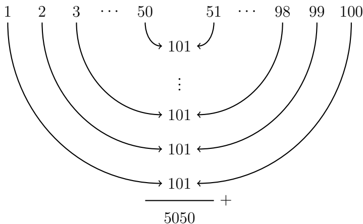
Obrázek 2.7: Gaussův trik pro sečtení prvních sto přirozených čísel.
