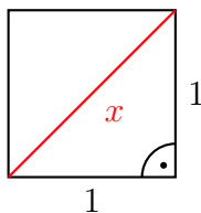
Obrázek 2.3: Čtverec o straně délky 1 a jeho úhlopříčka o straně délky x .
