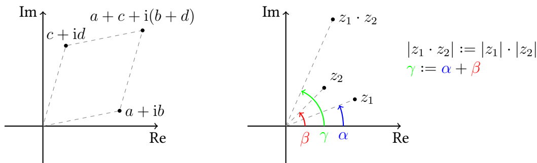
Obrázek 2.6: Geometrická interpretace operace sčítání a násobení komplexních čísel.
