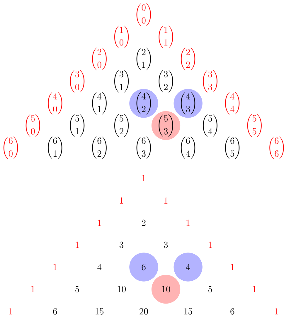
Obrázek 2.8: Pascalův trojúhelník.
