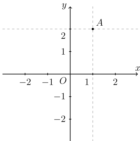
Obrázek 4.1: Pravoúhlý souřadný systém a bod A = (1, 2) .
