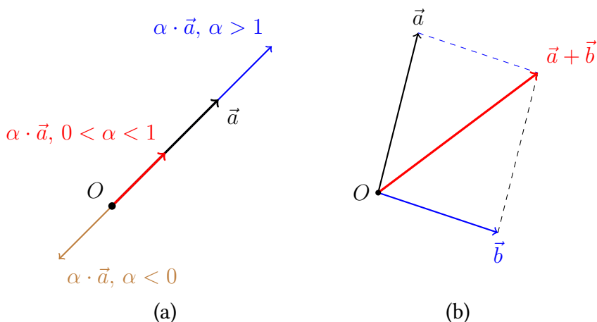
Obrázek 4.2: Geometrický význam násobení vektoru číslem (a) a sčítání vektorů (b).
