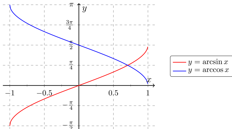
Obrázek 3.12: Grafy funkcí arcsin a arccos.
