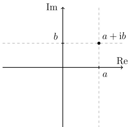
Obrázek 2.5: Komplexní rovina.
