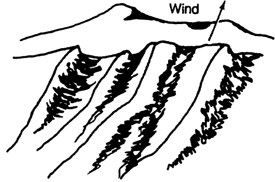
(b) Longitudinal
