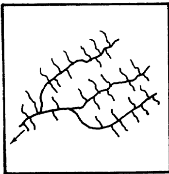
(d) Trellis
