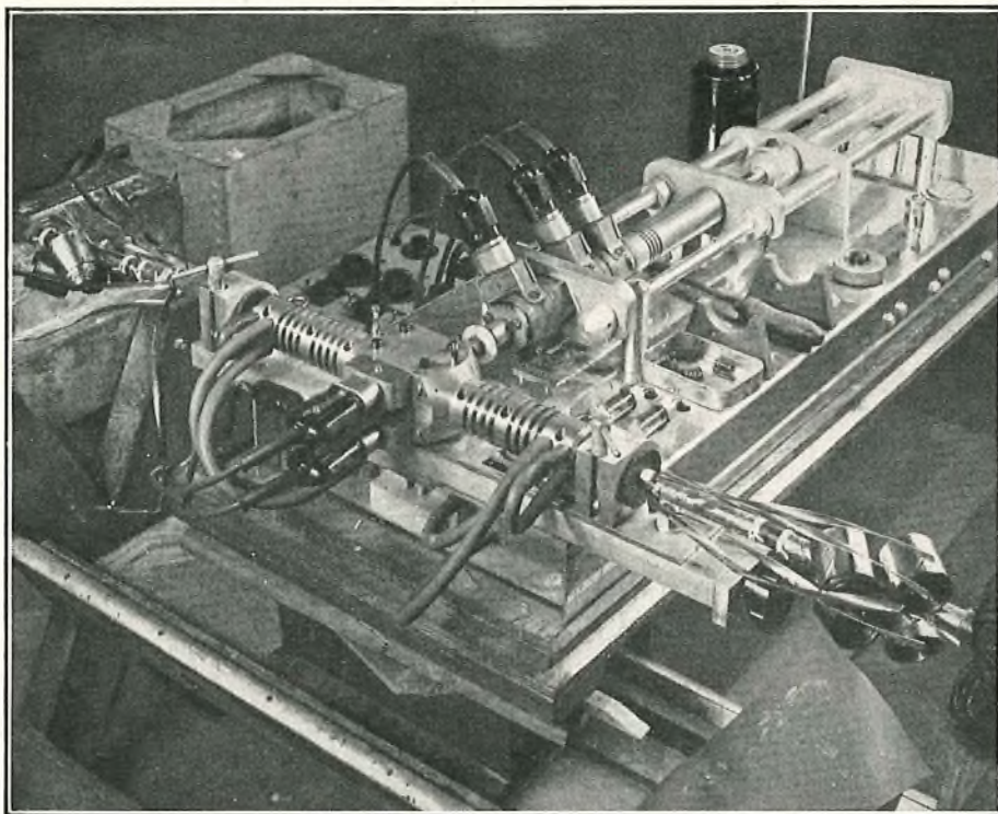
FIG. 3.—POLYTHENE-MOULDING MACHINE.
