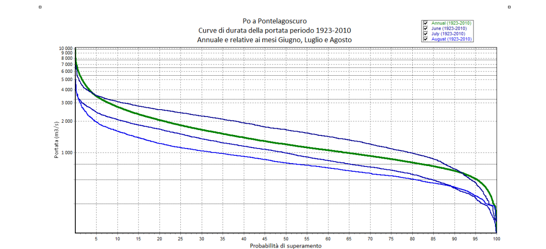
Figura 21 - Po a Pontelagoscuro - Curve di durata delle portate mensili per il periodo estivo, calcolate per il periodo 1923-2010. In verde è riportata la curva di durata annuale.
