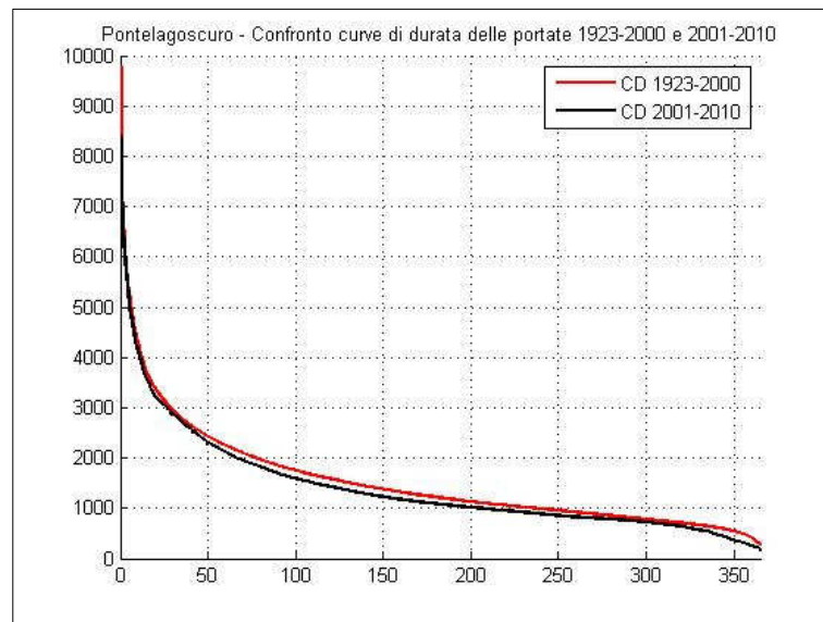
Figura 9 – Confronto tra la curva di durata riferita al periodo 1923-2000 e quella riferita all'ultimo decennio 2000-2010.
