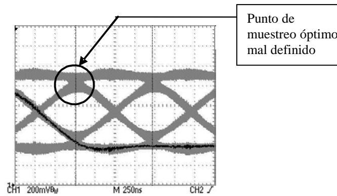
Figura 12-4. Diagrama en ojo con distorsión
