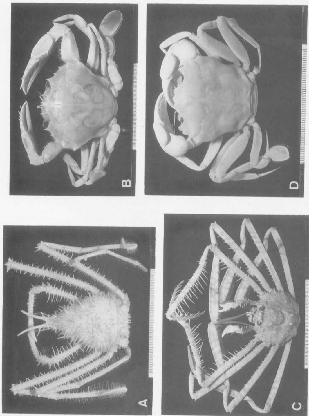
FIG. 14. A, Pleistacanthia oryx Ortmann, 1893, ♂, QM W10596; B, Ovalipes mollieri (Ward, 1933), ♀, QM W10564; C, Platyraia remifera Rathbun, 1916, ♂, QM W11240; D, Benthochascon hemingi Alcock and Anderson, 1899, ♂, QM W11236. Scale divisions 1 mm.
