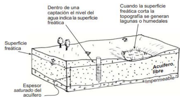
Figura 1. Acuífero no confinado o libre (Sánchez, 2011)
