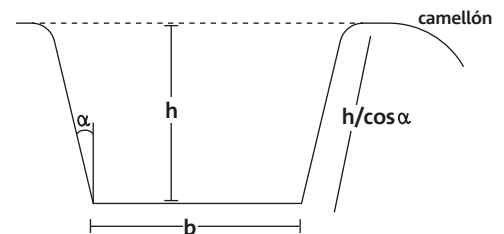
Configuración de un canal de desviación aguas lluvias
