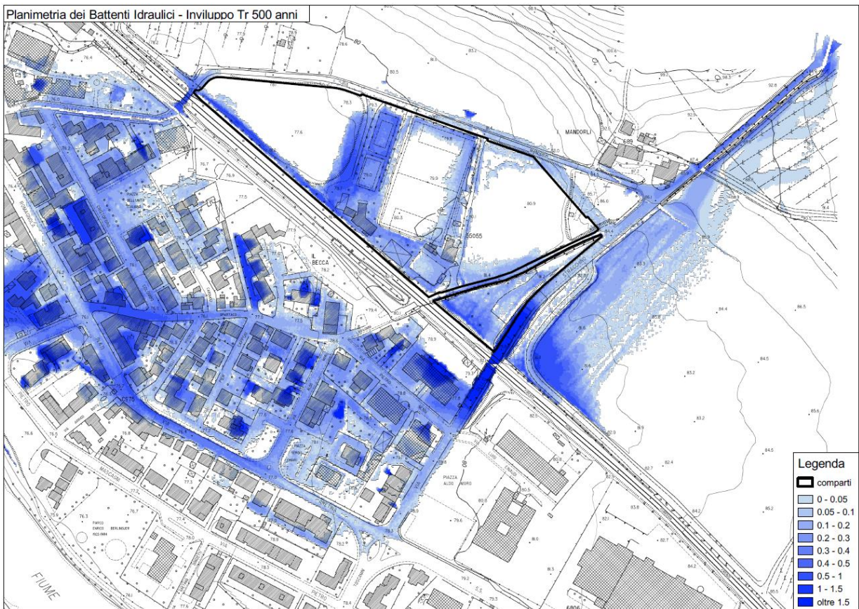
Figura 2-4: Inviluppo dei battenti idraulici TR 500 anni
