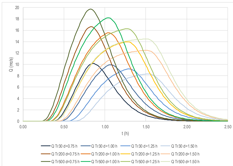
Figura 2-1: Idrogrammi di piena al variare del tempo di ritorno e della durata dell'evento meteorico ( m^3/s )
