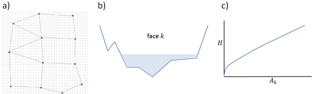
Figura 1: a) Esempio di “sotto-griglia”. b) Area bagnata associata ad una faccia della cella di calcolo k. c) Curva di invaso associata ad una cella di calcolo k.
