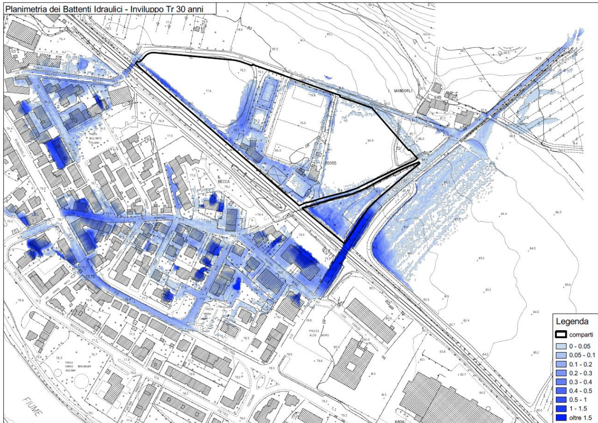
Figura 2-2: Inviluppo dei battenti idraulici TR 30 anni
