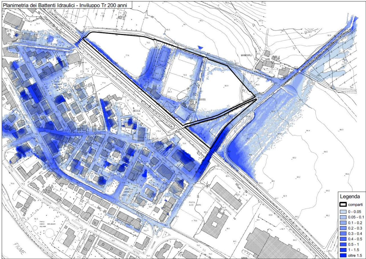
Figura 2-3: Inviluppo dei battenti idraulici TR 200 anni
