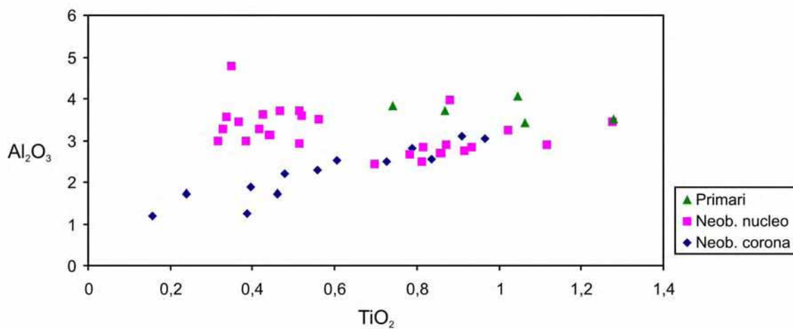
Fig. 3.4.4 – Variazioni composizionali di Al 2 O 3 vs TiO 2 per clinopirosseni magmatici (primari) e metamorfici (neoblasti) sin-Doc1 B . Per questi ultimi sono riportate le variazioni composizionali nucleo-corona.
