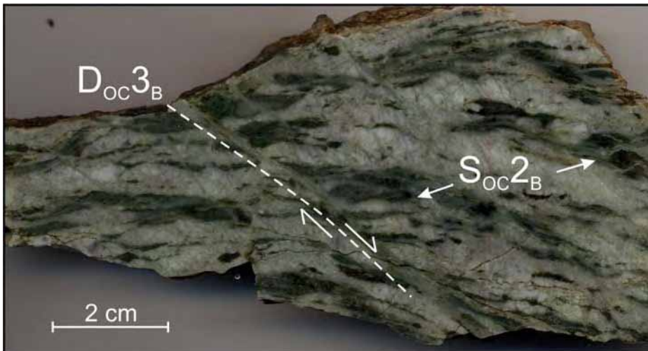
Fig. 3.3.2.25 – Zona di taglio (microfaglia) attribuita all'evento D_{OC3B} sviluppata all'interno di un meta-gabbro caratterizzato da una foliazione S_{OC2B} .
