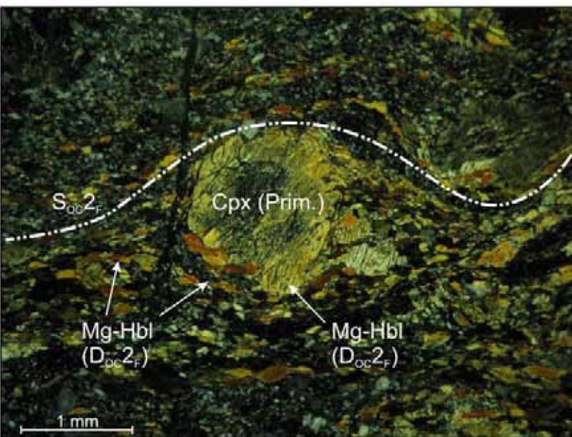
Fig. 5.2.1.4 – Mg-orneblenda pseudomorfa su un porfiroclasto di clinopirosseno primario. La deformazione D_{OC2F} determina lo sviluppo sin-cinematico di anfiboli analoghi nelle code di pressione (microfoto, nicols + ).
