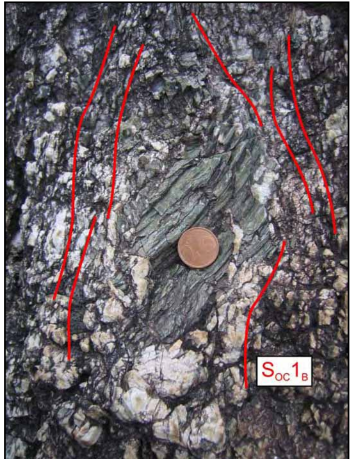
Fig. 3.3.2.7 – Porzione di gabbro a tessitura pegmatoide preservata dalla deformazione metamorfica ( D_{OC1_B} ), concentrata nei volumi di roccia (caratterizzati da una tessitura primaria più fine) limitrofi.
