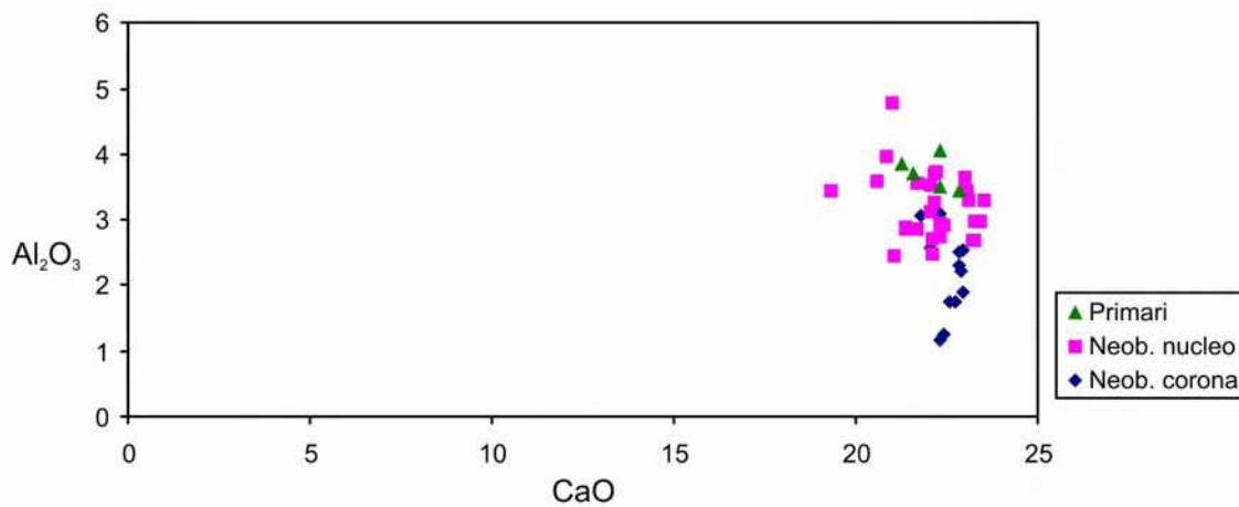
Fig. 3.4.3 – Variazioni composizionali di CaO vs Al 2 O 3 per clinopirosseni magmatici (primari) e metamorfici (neoblasti) sin-Doc1 B . Per questi ultimi sono riportate le variazioni composizionali nucleo-corona.
