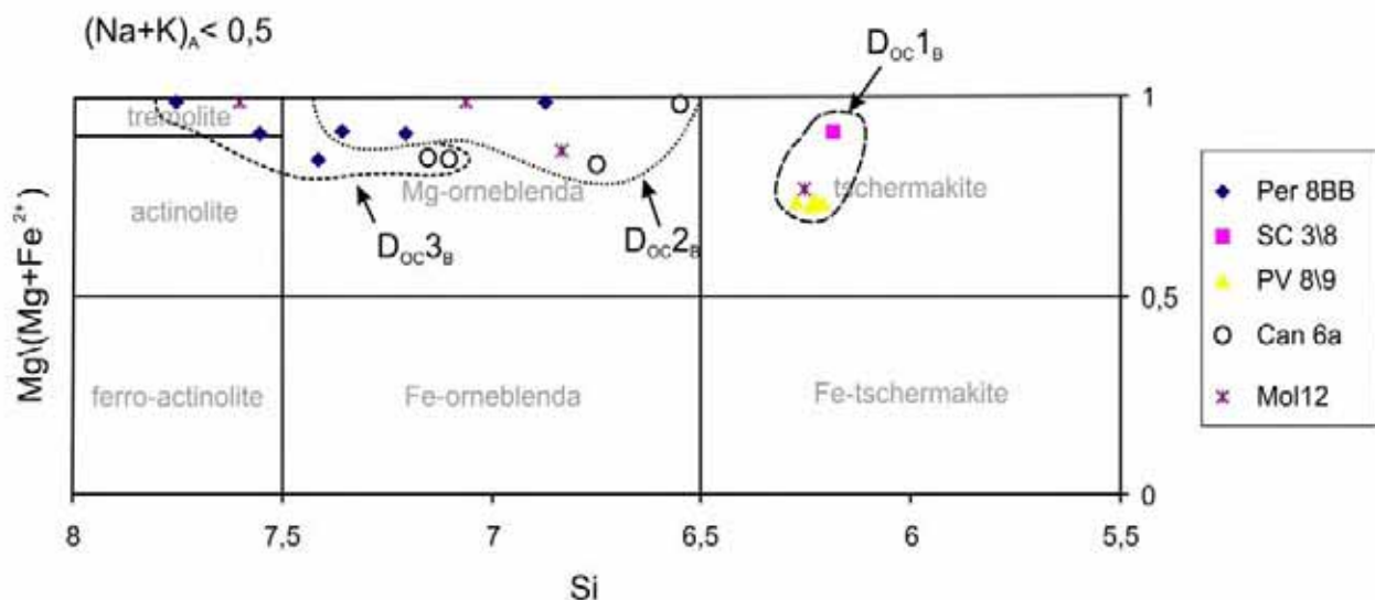
Fig. 3.4.9 – Composizione degli anfiboli calcici secondo Leake et al., 1997.
