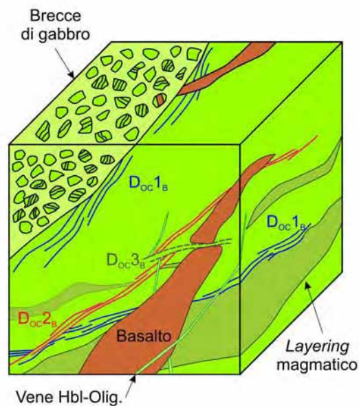
Fig. 6.1.1.2 – Relazioni di interferenza tra le diverse fasi metamorfico\deformative riconosciute all'interno del complesso gabbrico.
