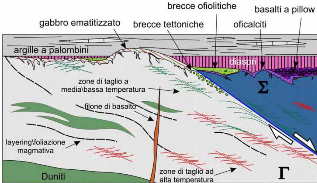
Fig. 6.4.2 – Sezione schematica riassuntiva proposta per l'evoluzione e l'esumazione oceanica dei complessi gabbrici "tipo-Bracco" (Γ- gabbro, Σ-peridotiti).
