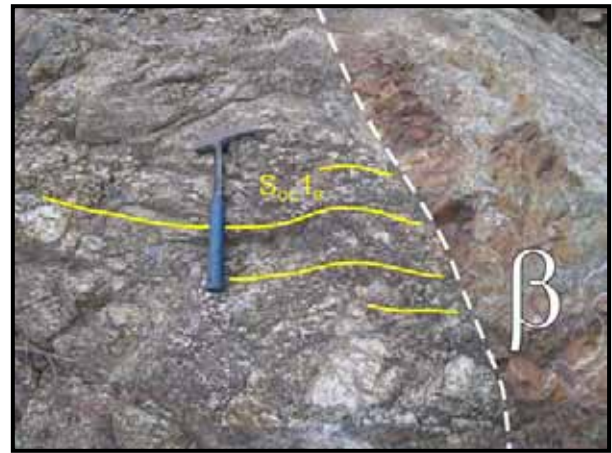
Fig. 3.3.2.20 – Relazione di interferenza tra un filone di basalto ( \beta ) e la foliazione S_{OC1B} .
