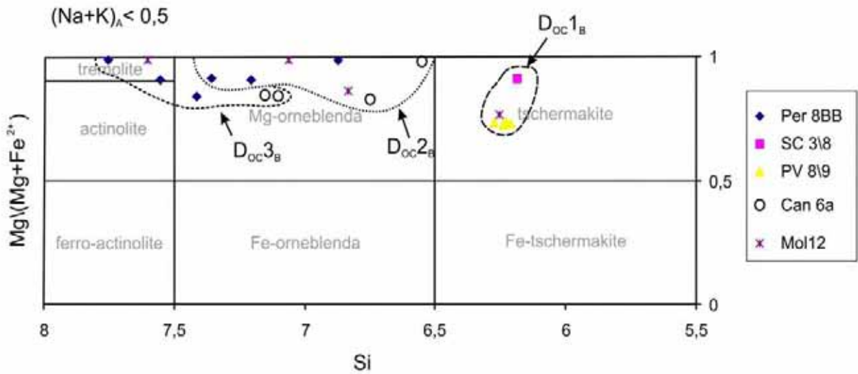
Fig. 3.4.10 – Composizione degli anfibi calcici secondo Leake et al., 1997.
