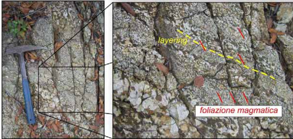
Fig. 3.3.1.1 – Relazione di interferenza tra la foliazione magmatica, costituita da allineamenti di pirosseni e plagioclasì, ed il layering magmatico (Loc. Sciona).
