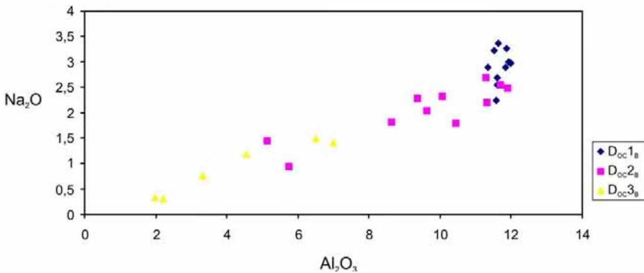
Fig. 3.4.12 – Variazioni composizionali di Na_2O vs Al_2O_3 per anfibi, in relazione alla fase metamorfica di appartenenza.
