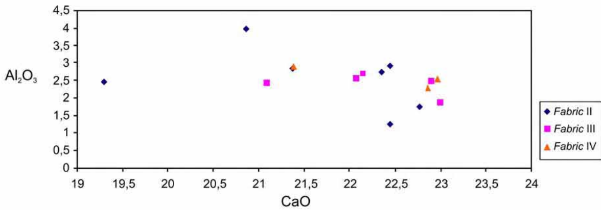
Fig. 3.4.5 – Variazioni composizionali di CaO vs Al 2 O 3 per clinopiroseni metamorfici sin-D OC 1 B , relativi a diversi termini del fabric in uno stesso campione (PV8\9).
