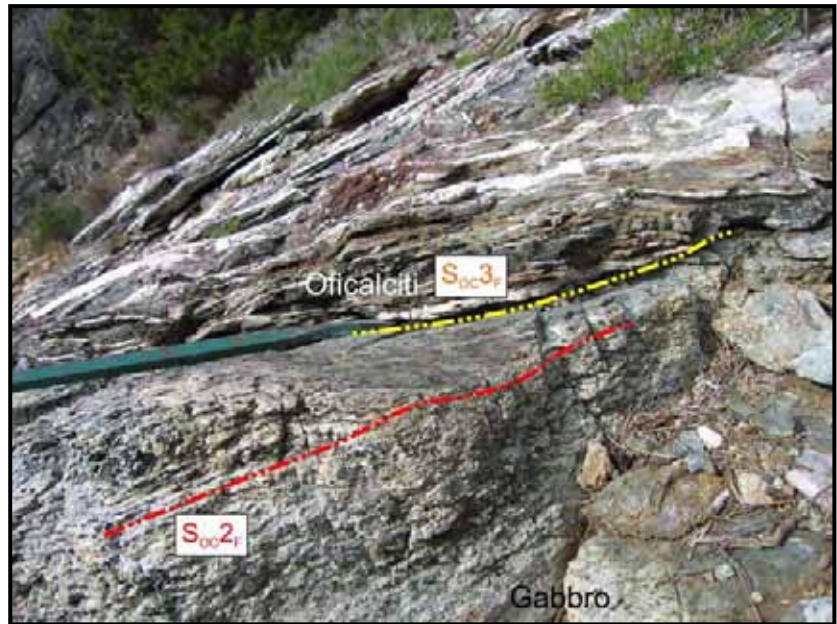
Fig. 5.2.1.3 – Superficie di contatto tra il gabbro e le oficalciti: la foliazione S_{OC2F} risulta sub-parallela all'interfaccia tra le due litologie ed alla S_{OC3F} .
