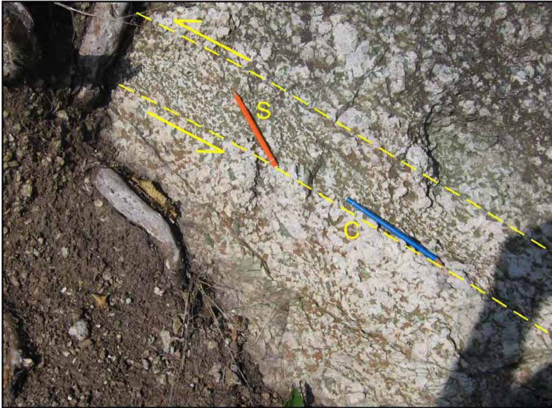
Fig. 3.3.1.4 – Zona di taglio S-C sin-magmatica (Loc. Pietra di Vasca).
