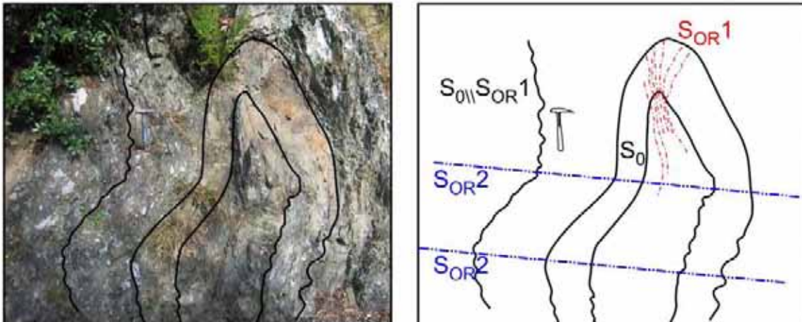
Fig. 3.6.8 – Piega isoclinal di prima fase F_{OR1} deformata da una piega di seconda fase F_{OR2} .
