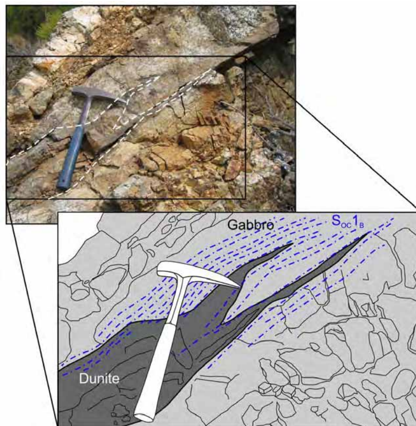
Fig. 3.3.2.1 – Shear zone ( D_{oc1B} ) sviluppata all'interfaccia dunitelgabbro. I rapporti tra i due litotipi risultano trasposti dalla deformazione metamorfica (loc. Moggia-Pian della Madonna).
