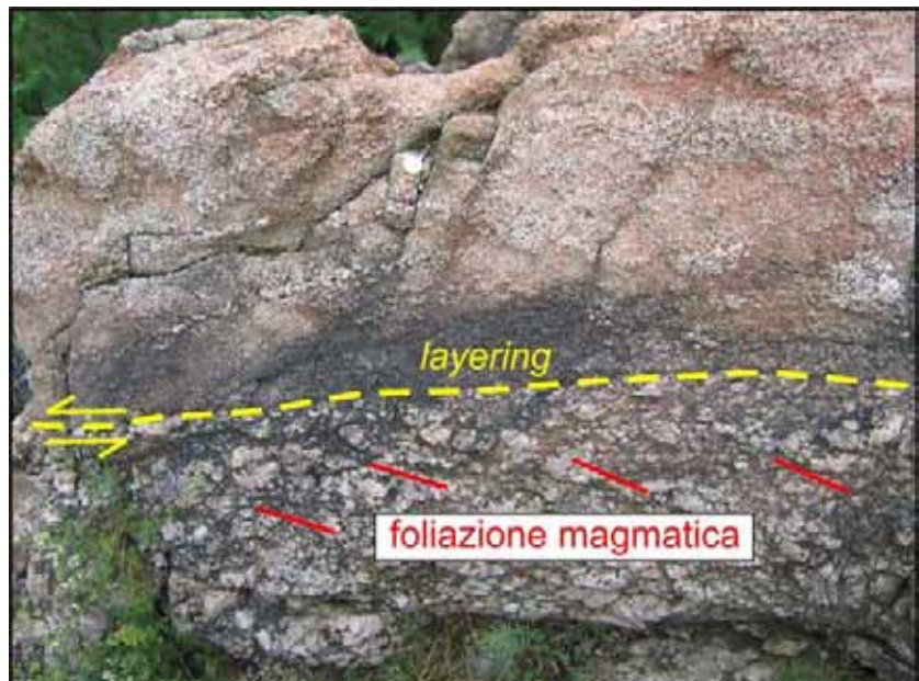
Fig. 3.3.1.2 – Discordanza angolare, con geometria S-C, tra la foliazione magmatica, costituita da livelli "nastri" di plagioclasio, ed il layering magmatico (Loc. Sciona).
