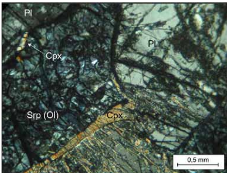
Fig. 3.2.2.2 – Gabbo olivinico: clinopirosseno pecilitico sviluppato nell'interfaccia olivina-plagioclasio (microfoto, nicols + ).
