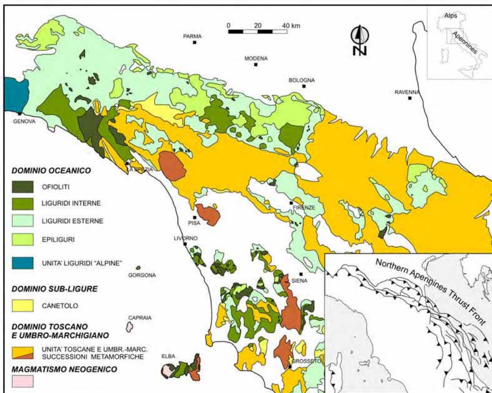
Fig. 2.1.1 – Carta tettonica schematica dell'Appennino Settentrionale (tratta e modificata da Principi et al., 2004 cum bibl. ).
