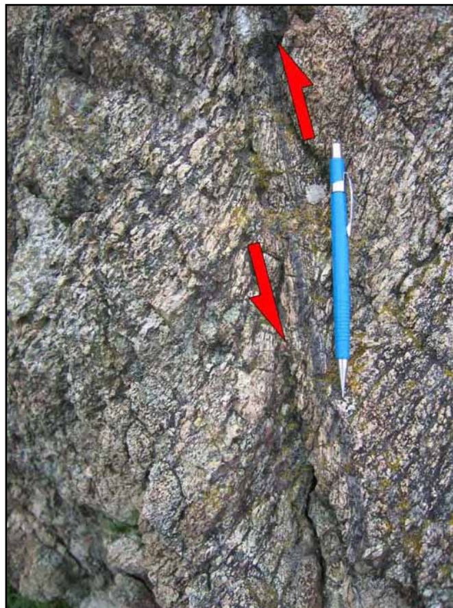
Fig. 3.3.2.3 – Zona di taglio milonitica D_{OC1B} all'interno di gabbri. Il senso movimento è desunto in maniera univoca dalle asimmetrie della foliazione metamorfica.
