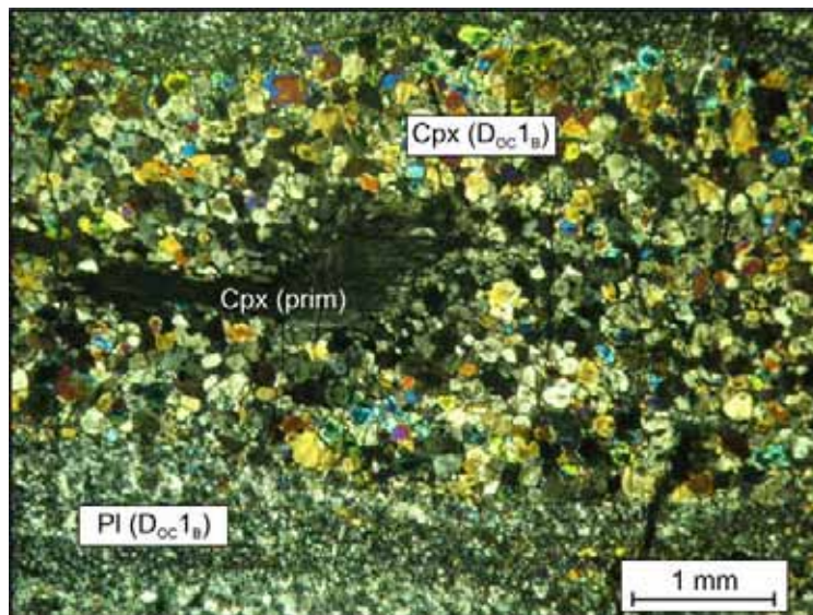
Fig. 3.3.2.14 – Fabric II: relitto di clinopirosseno magmatico-primario circondato da una corona di clinopirosseni neoformati ( sin-D oc1B ). I plagioclasii primari sono sostituiti completamente da aggregati granoblastici di plagioclasii sin-D oc1B (microfoto, nicois + ).
