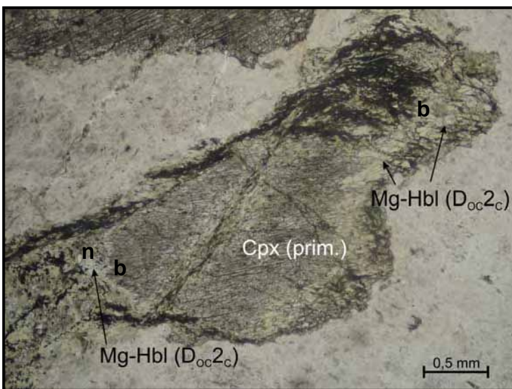
Fig. 4.2.4 – Mg-orneblende (sin- D_{oc}2_c ) da brune (b) ad incolore (n) sviluppate dinamicamente intorno ad un clinopirosseno primario (microfoto, nicols \).
