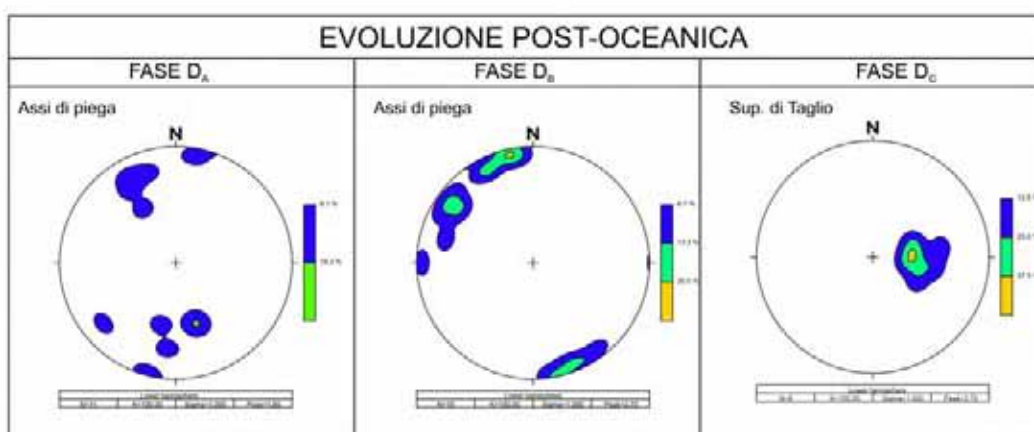
TAV. I Fet - Diagrammi stereografici relativi all'orientazione delle strutture metamorfiche riconosciute nell'area di Punta Fetovaia. Per i piani sono rappresentati i poli (reticolo di Schmidt, emisfero inferiore).
