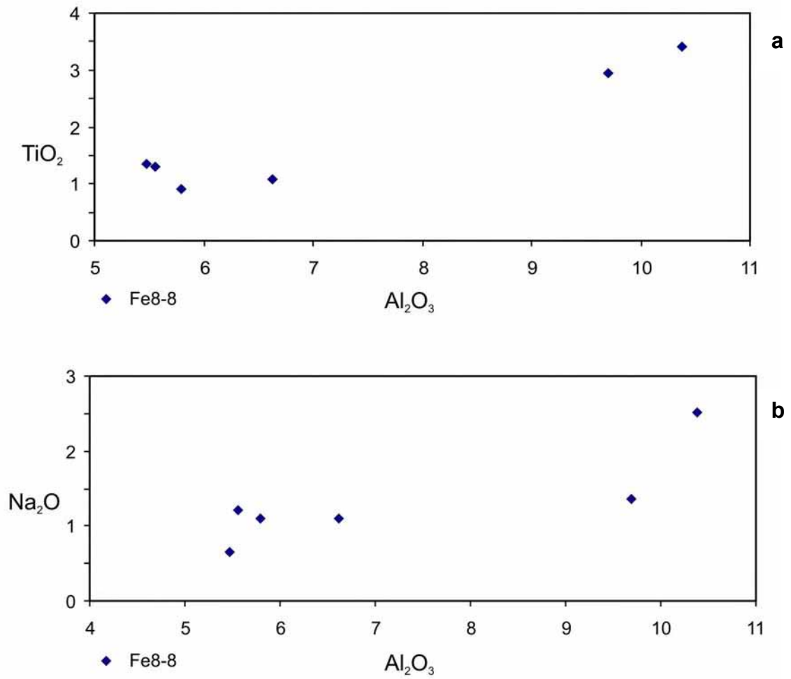
Fig. 5.3.3 – Variazioni composizionali di TiO 2 vs Al 2 O 3 (a) e Na 2 O vs Al 2 O 3 (b) per anfiboli metamorfici (D 0c2F ).
