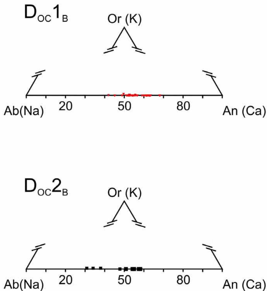
Fig. 3.4.7 – Composizione dei plagioclasi in relazione alla fase metamorfico\deformativa.
