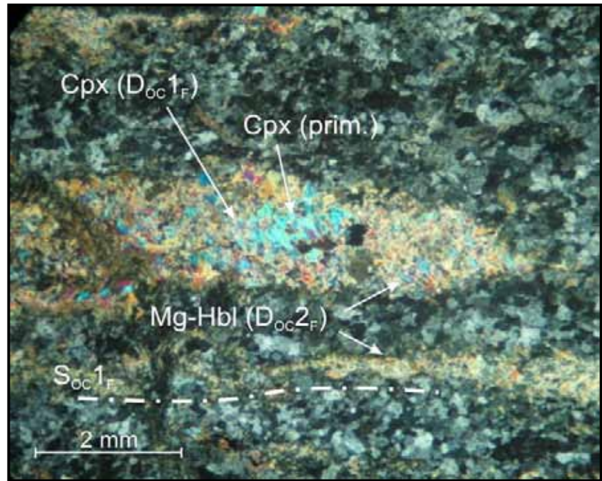
Fig. 5.2.1.2 – Relitti tessuturali di Cpx primari e sin-D_{OC1F} circondati da aggregati di anfiboli (Mg-orneblenda) cristallizzati staticamente (microfoto, nicols +).
