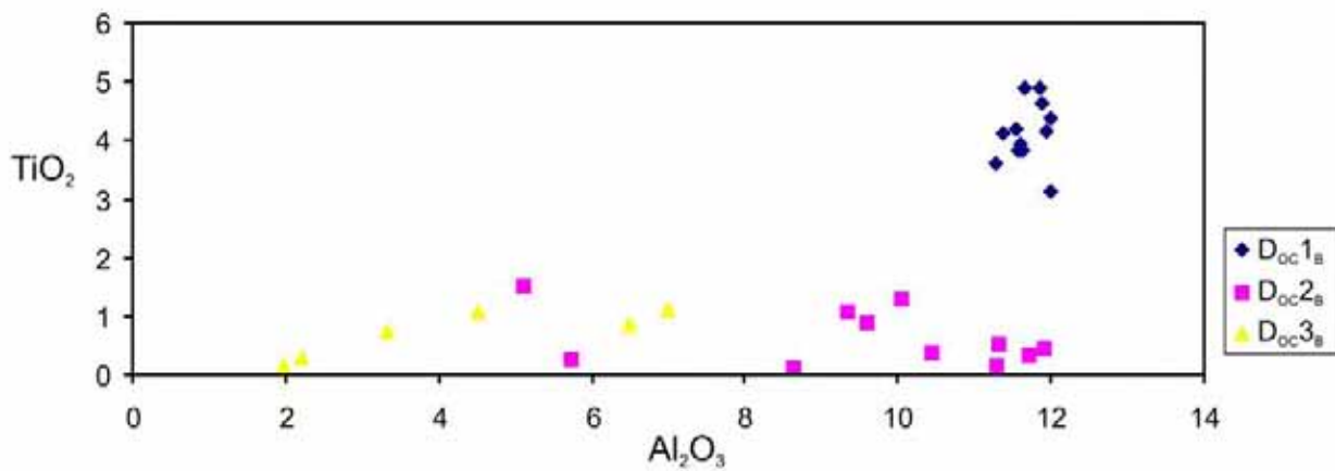
Fig. 3.4.11 – Variazioni composizionali di TiO_2 vs Al_2O_3 per anfibi, in relazione alla fase metamorfica di appartenenza.
