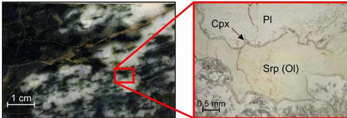
Fig. 3.3.1.6 – Foliazione magmatica. Nell'ingrandimento: clinopiroseno pecilitico primario, indeformato, sviluppato intorno ad olivina primaria serpentinizzata (microfoto, nico/s \).
