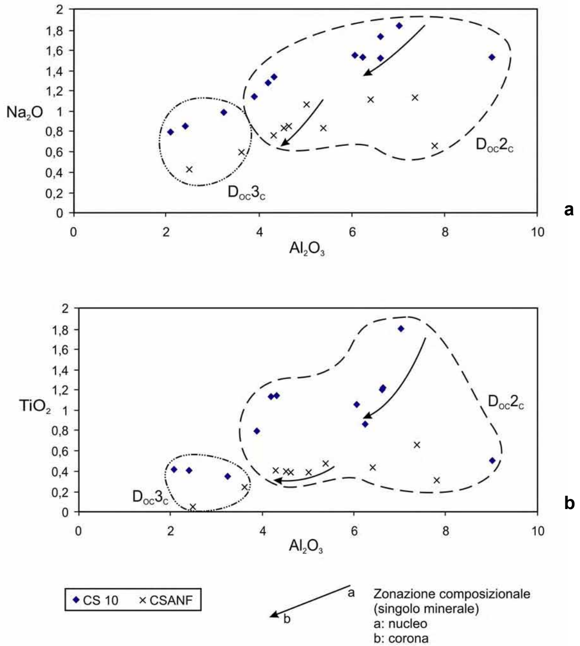
Fig. 4.3.5 – Variazioni composizionali di Na 2 O vs Al 2 O 3 (a) e TiO 2 vs Al 2 O 3 (b) per anfiboli metamorfici.
