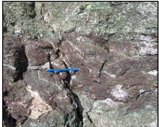
Fig. 3.1.2.3 – Superfici arrossate ed ematizzate all'interno dei gabbri.
