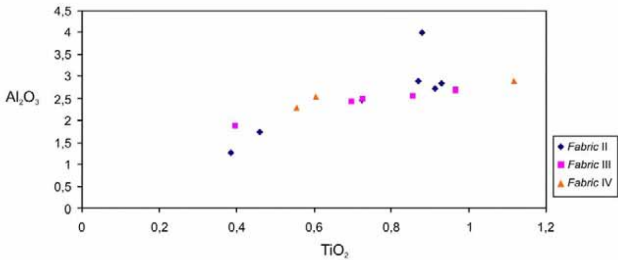
Fig. 3.4.6 – Variazioni composizionali di TiO 2 vs Al 2 O 3 per clinopiroseni metamorfici sin-D OC 1 B , relativi a diversi termini del fabric in uno stesso campione (PV8\9).
