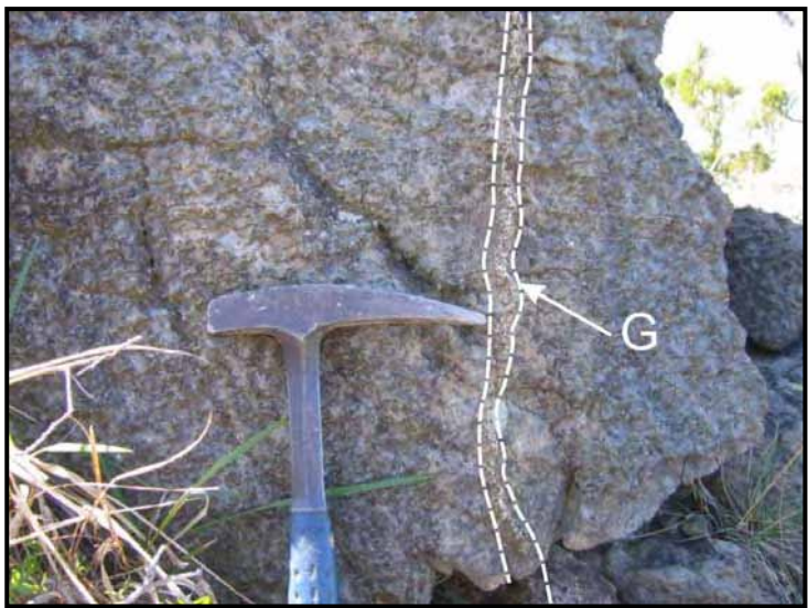
Fig. 3.1.1.3 - Filone gabbrico (G) intruso dentro delle peridotiti Iherzolitiche.
