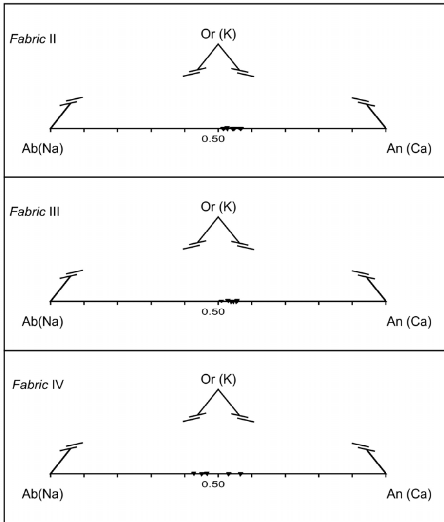
Fig. 3.4.8 – Variazione composizionale dei plagioclasti sin-D 0c1B relativi a diversi termini del fabric in uno stesso campione (PV819).
