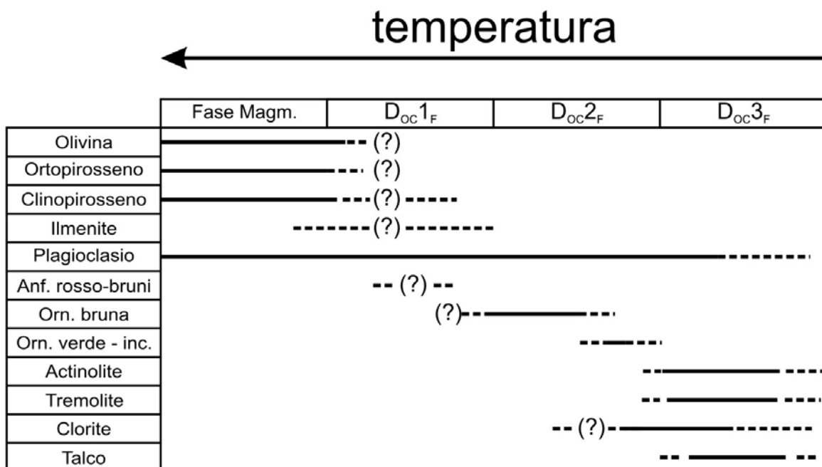
Fig. 6.3.1.2 – Tabella riassuntiva relativa ai rapporti di blastesi-deformazione ricostruiti per l'evoluzione metamorfo oceanica dei gabbri di Punta Fetovaia.
