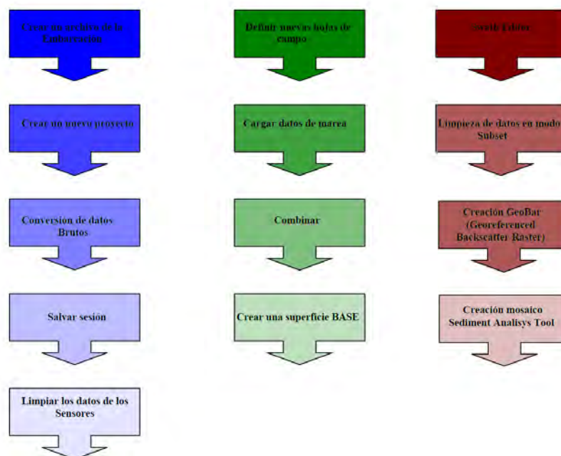
Figura 4.3. - Flujo de trabajo en el entorno de Caris HIPS and SIPS para el procesado de la reflectividad obtenida con ecosonda multihaz.
