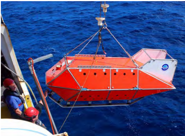
Figura 4.10.5.- Largando el trineo de fotogrametría TFS-2 desde el pórtico de hidrografía del B/O Thalassa . Pantalla del programa de control de vuelo y registro de datos en tiempo real.
