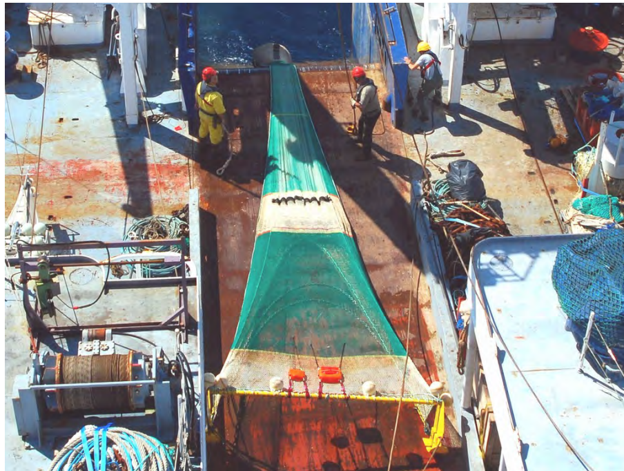
Figura 4.5.4.- Recuperando el bou de vara a bordo del B/O Thalassa durante la campaña INDEMARES 0710. Se pueden observar los sensores Scanmar en la parte superior del aparejo para monitorizar la unidad de muestreo.
