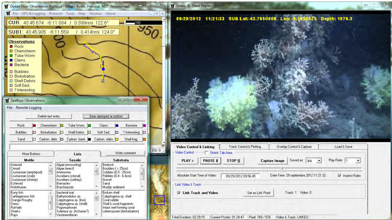
Figura 4.10.11. Interface del programa OFOP de integración de la telemetría, observaciones y vídeo utilizado para la monitorización de los transectos visuales directos con los vehículos submarinos Liropus y Pollitolana .
