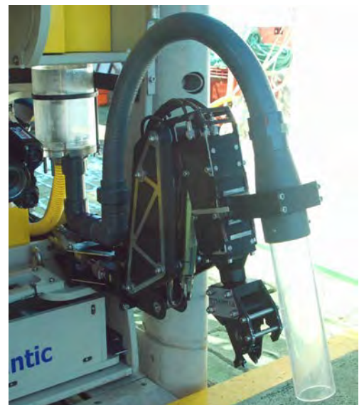
Figura 4.10.2.- A) Brazo manipulador de 6 grados de libertad Hydrolek HLK-47000 (a la izquierda) para la captura de ejemplares vivos y B) sistema de succión acoplado al manipulador Hydrolek HLK-HD45 de 5 funciones (a la derecha).
