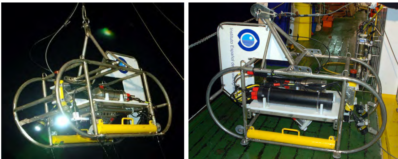
Figura 4.10.4. Operaciones nocturnas con el trineo Politolana durante la campaña A0412. Se puede observar la disposición de los focos DSPL Sphere (foto izquierda) y del multiplexador NEXUS MKE (foto derecha).
