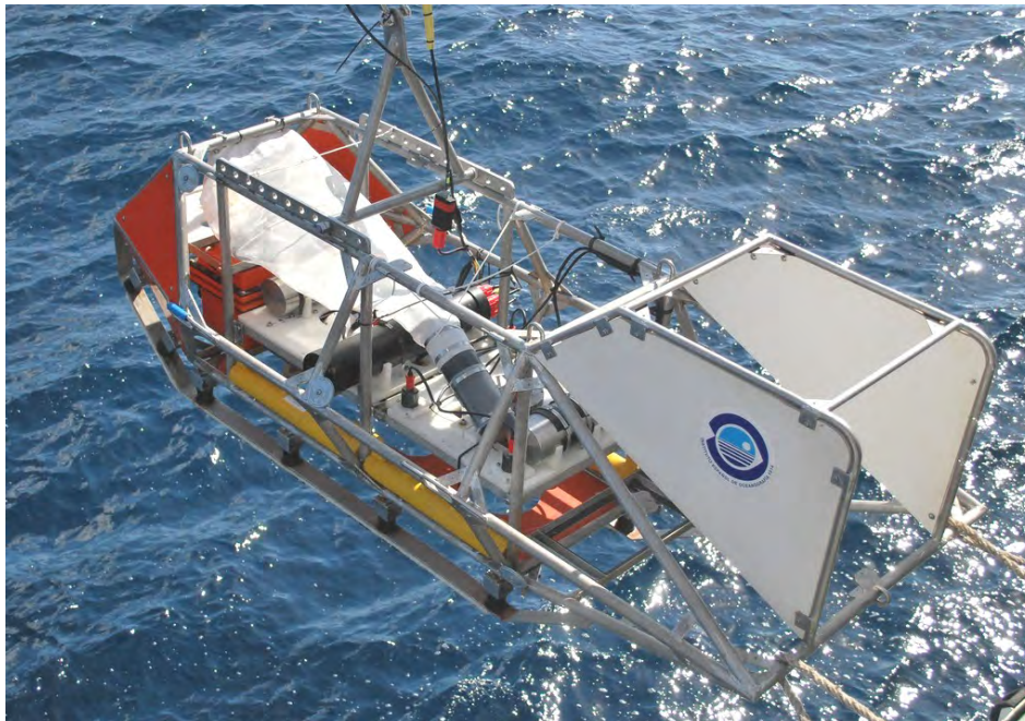
Figura 4.10.6.- Trineo fotogramétrico TFS-2 durante la campaña A0912. Se puede observar la disposición de la red para la captura de organismos suprabentónicos sobre hábitats de fondos duros tridimensionalmente complejos.
