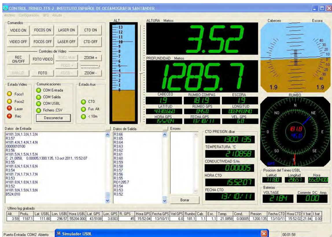
Figura 4.10.10. Interface del programa de control de vuelo (versión 2012) de los trineos TFS-2 y Pollitolana que integra y sincroniza la telemetría de los diferentes subsistemas para la monitorización de los transectos visuales directos con los vehículos submarinos. En la tabla inferior con encabezado “Ultimo log grabado” se muestran los parámetros archivados cada segundo.
