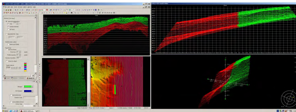
Figura 4.3.6.- Interfaz que ofrece la aplicación informática Caris HIPS and SIPS para la limpieza de las sondas obtenidas con ecosonda multihaz, a través del editor de bandas de sondaje.
