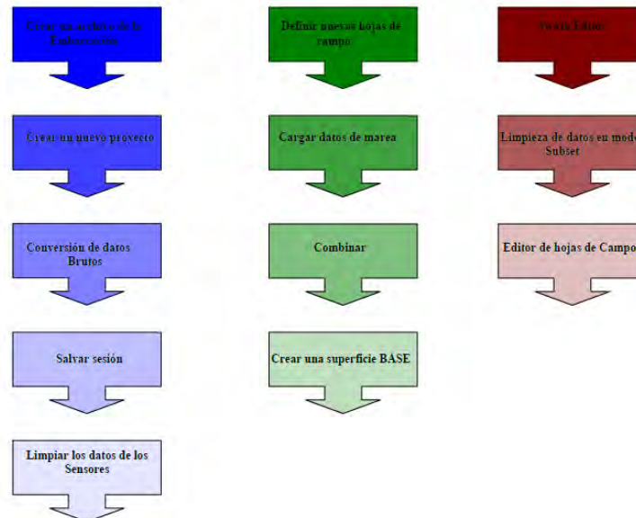
Figura 4.3.5.- Flujo de trabajo en el entorno de Caris HIPS and SIPS para el procesado de las sondas obtenidas con ecosonda multihaz.
