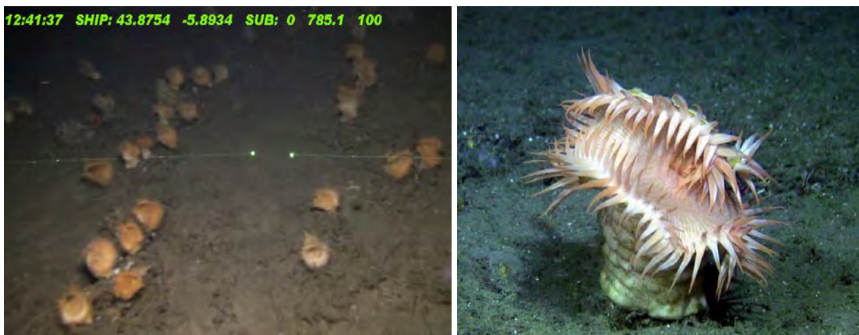
Figura 1.11.- Facies y especies características de los fondos detríticos de cañones submarinos: A) valle del cañón del Corbiro a 785 m y B) detalle de la anémona Phelliactis hertwigi .
