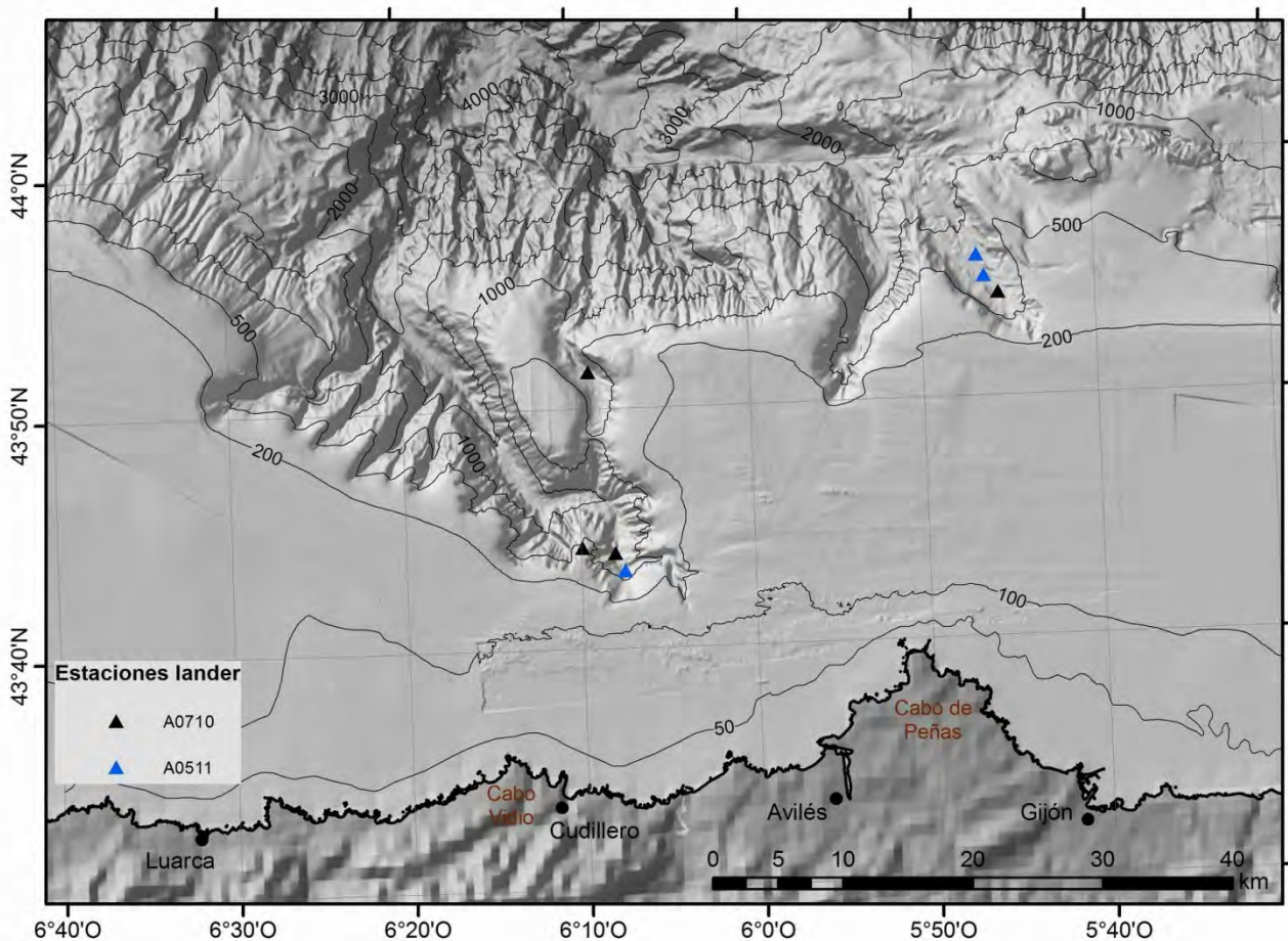
Figura 4.10. .- Situación de los fondeos con el lander efectuados durante las campañas INDEMARES.
