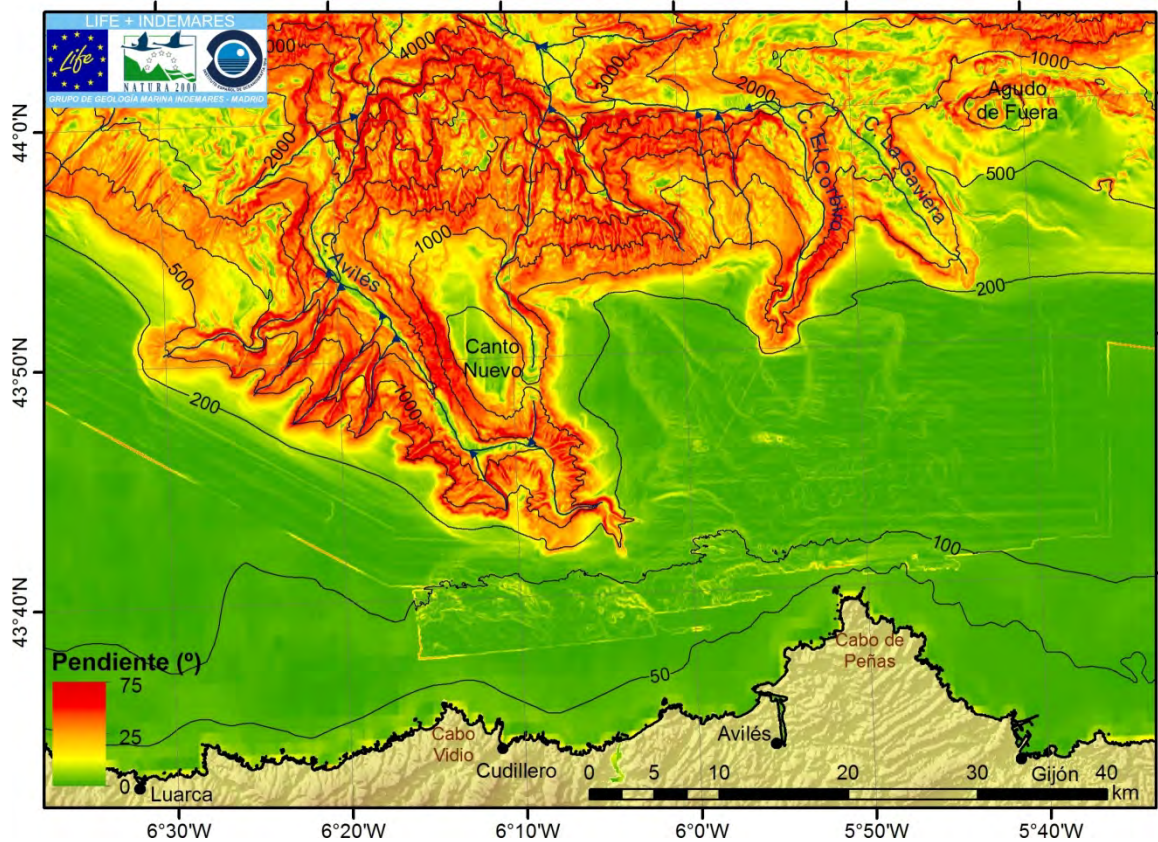
Figura 5.2.2.- Panel superior: Modelo digital del terreno del área de estudio, codificado en color. Iluminación desde el NO. Panel inferior: Modelo de pendientes del área de estudio, codificado en color y con algunos contornos batimétricos superpuestos.
