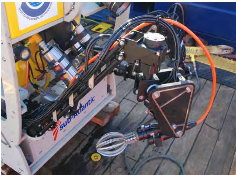
Figura 4.10.2.- A) Brazo manipulador de 6 grados de libertad Hydrolek HLK-47000 (a la izquierda) para la captura de ejemplares vivos y B) sistema de succión acoplado al manipulador Hydrolek HLK-HD45 de 5 funciones (a la derecha).
