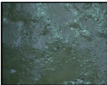
Figura 5.2. .- Fotografías de la superficie del sedimento y curvas granulométricas de dos de las estaciones muestreadas en el estrato de 500 a 1000 m de profundidad (una estación con alto contenido en arena gruesa, VI, y otra estación con alto contenido en fango, XIII).
