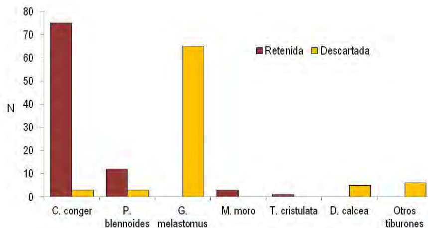
Figura .2.2 .- Especies capturadas y retenidas en un embarque de palangre de fondo dirigido al congrio en poca profundidad.
