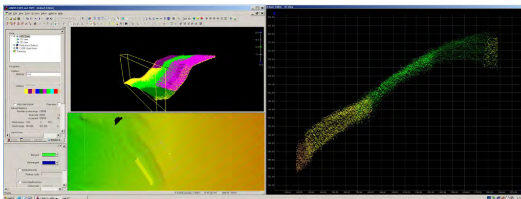
Figura 4.3. - Interfaz que ofrece la aplicación informática Caris HIPS and SIPS para la limpieza de las sondas obtenidas con ecosonda multihaz, en este caso, a través del editor de subconjuntos de datos, especialmente indicado para el control del solape entre líneas.
