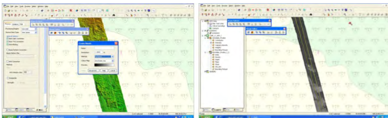
Figura 4.3.10.- Interfaz que ofrece la aplicación informática Caris HIPS and SIPS para creación de un mosaico de reflectividad con el módulo Geocoder.
