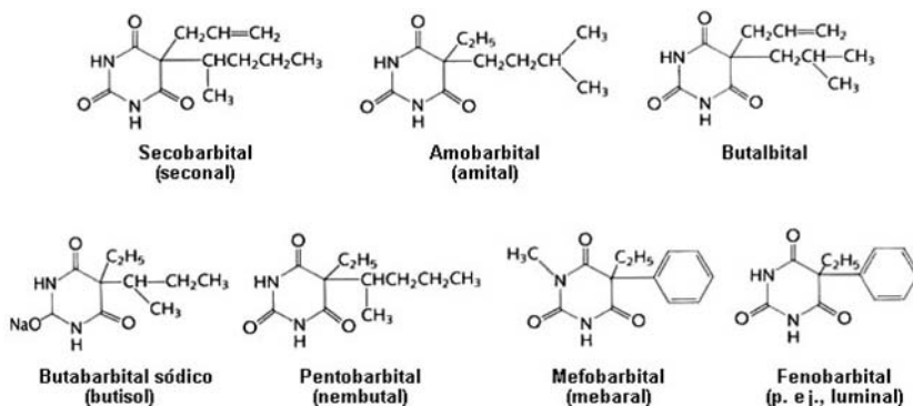
Figura 17. Estructura química de algunas de las sustancias de naturaleza barbitúrica sintetizadas.
