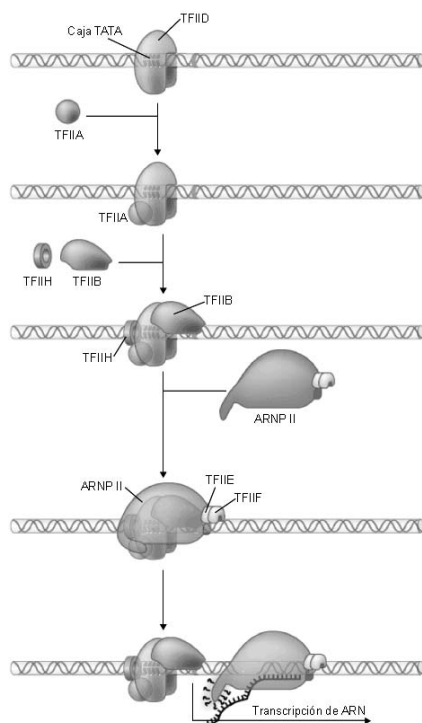
Figura 17. Interacciones con la zona promotora. Fuente: Hodge, 2009.
