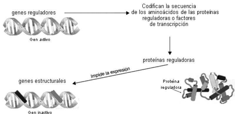
Figura 2. Regulación de la expresión génica en el ámbito transcripcional mediante proteínas reguladoras. Para ello, se unen de forma selectiva a una región específica del ADN situada al inicio de los genes estructurales (secuencia reguladora) impidiendo la unión de la ARN polimerasa, y por tanto, la expresión del gen estructural.
