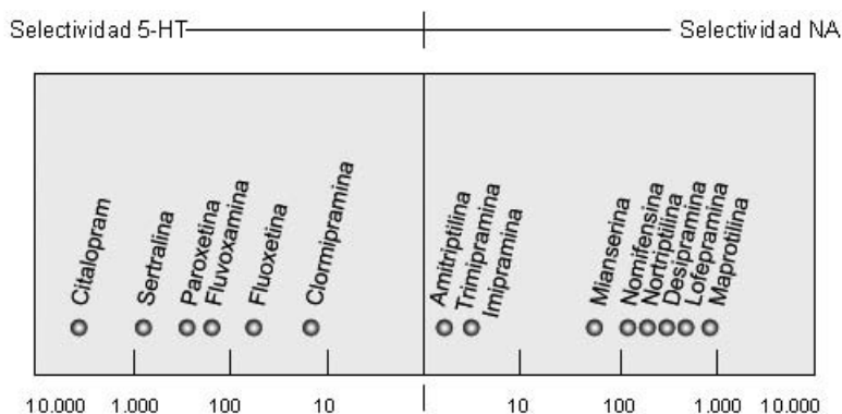
Figura 16. Cocientes de selectividad de distintos inhibidores de recaptación determinados in vitro . Los fármacos situados más hacia la izquierda son más selectivos para la inhibición de la recaptación de 5-HT, mientras que los situados a la derecha lo son para la NA.
