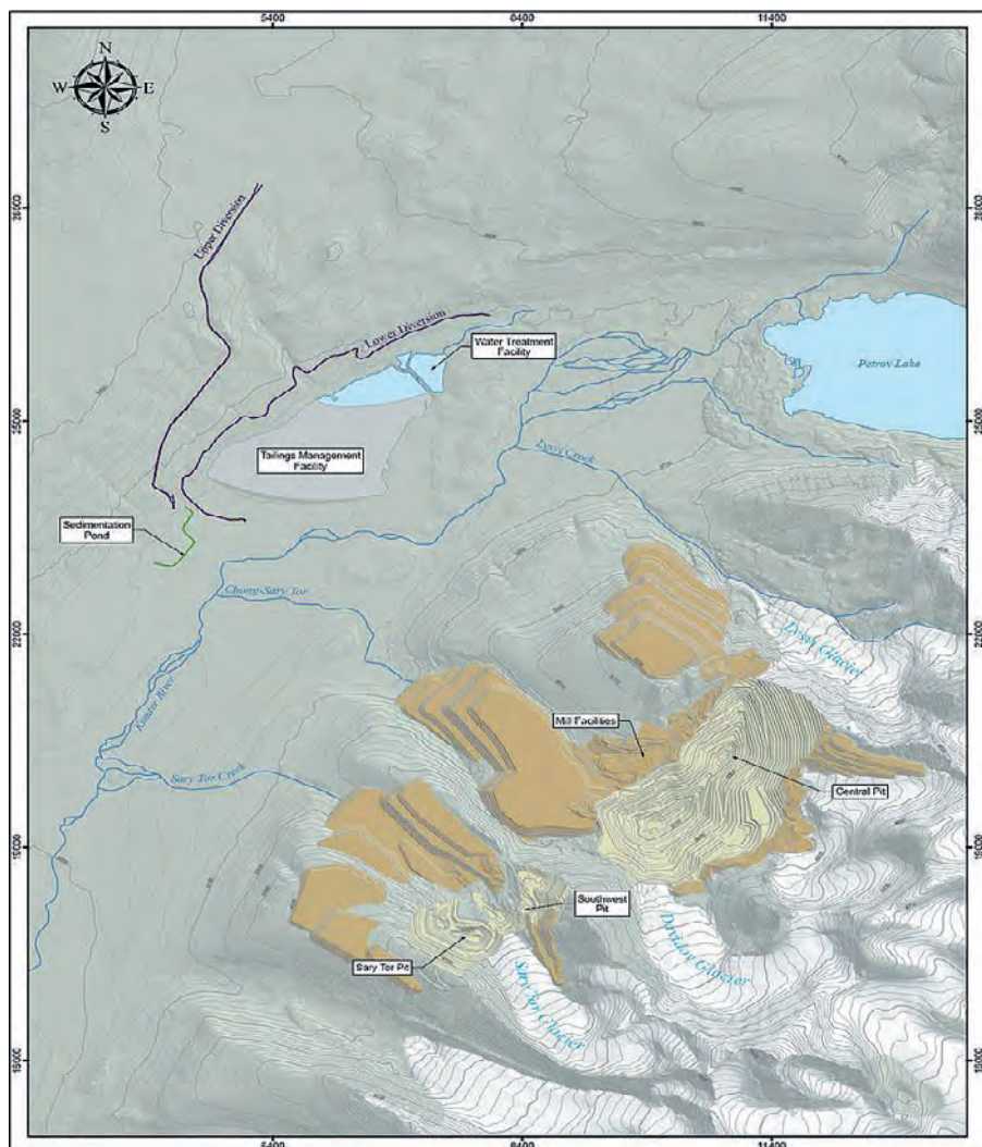
Схема 9-1: Схема размещения отвалов
