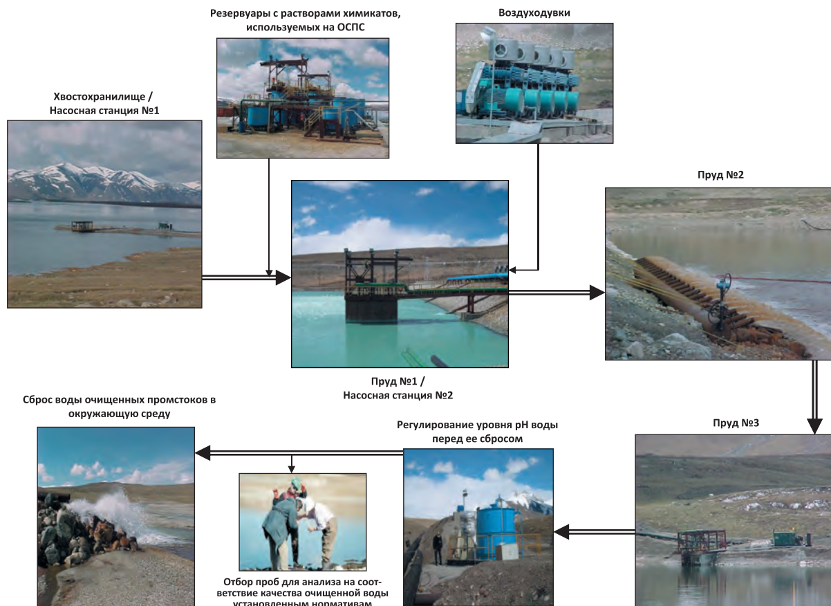
Схема 8-4: Схема технологии очистки промстоков
