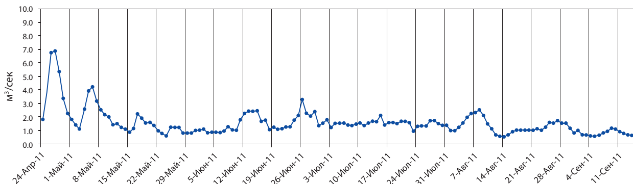
Диаграмма 6-16: Гидрометрический мониторинг верхнего отводного канала
