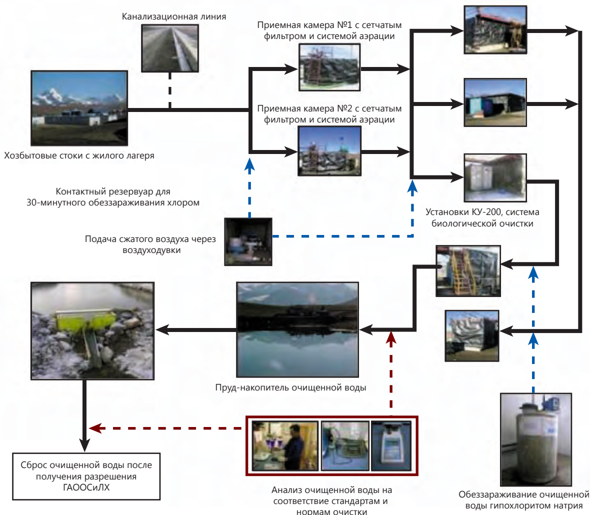
Схема 8-2: Схема технологии очистки хозяйственных стоков
