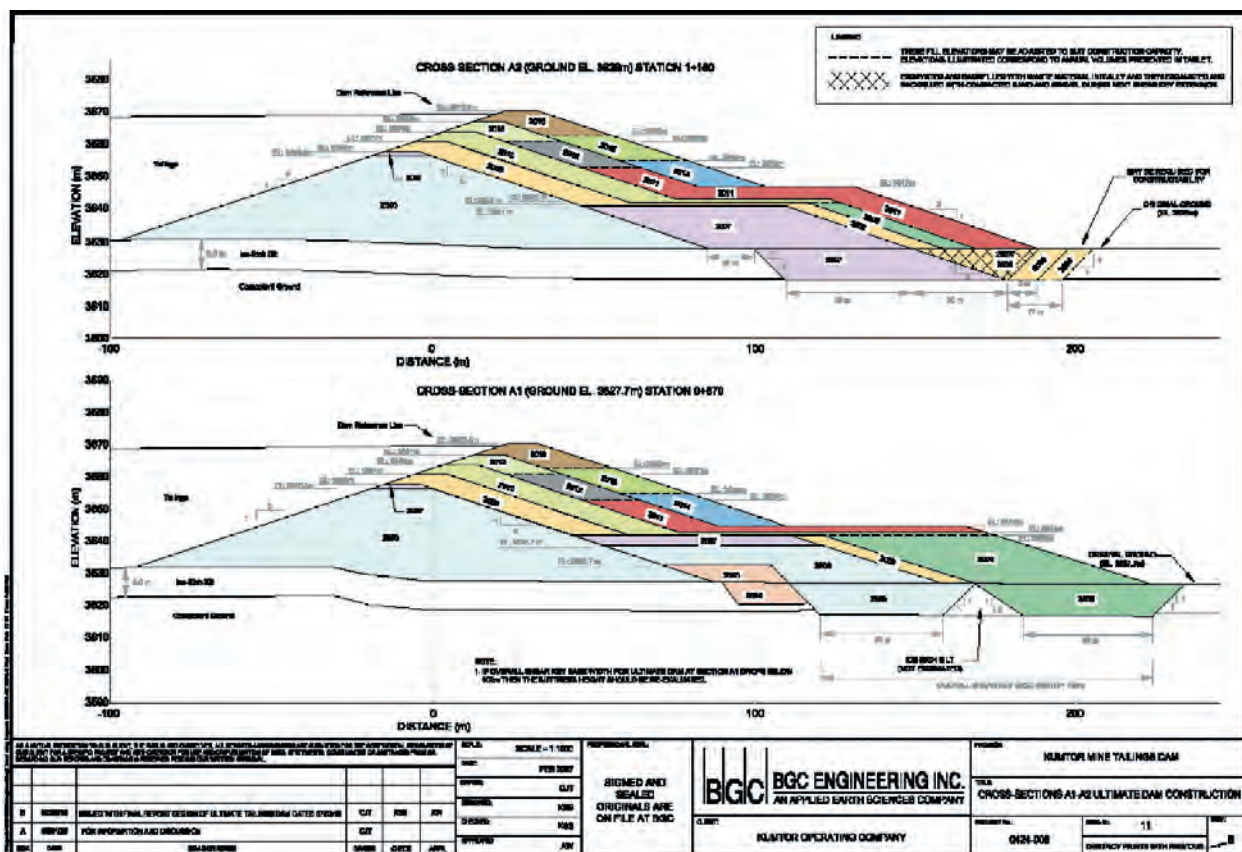
Схема 8-1: Нарращивание дамбы хвостохранилища
