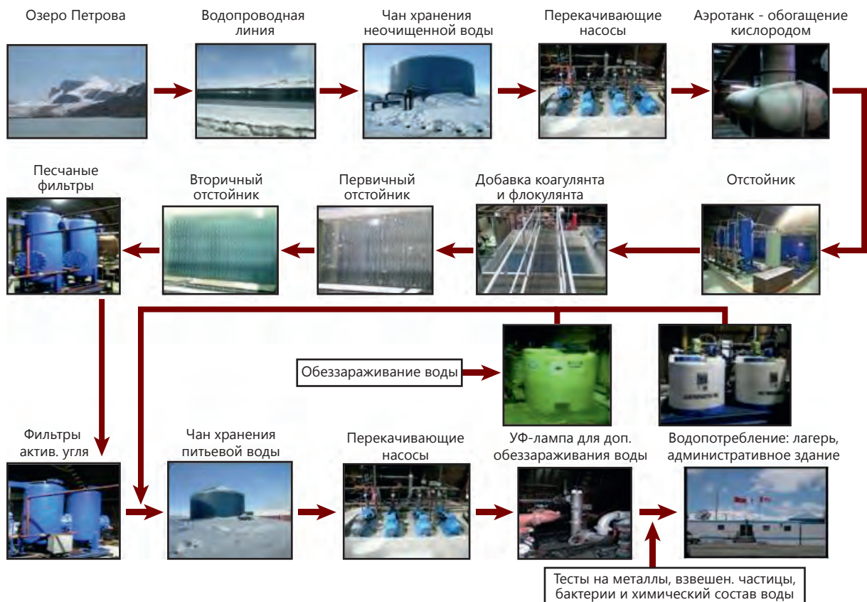
Схема 8-3: Схема технологии очистки питьевой воды на СОПВ (нижняя зона рудника)
