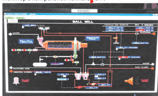
Монитор в контрольной комнате ЗИФ
