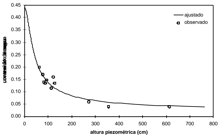
Figura 1: curva de retención ajustada por el modelo de van Genuchten.
