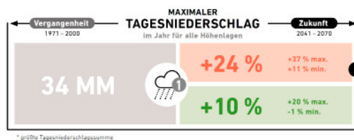
Prognose maximaler Tagesniederschlag. © ZAMG
