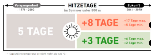
Prognose Hitzetage. © ZAMG
