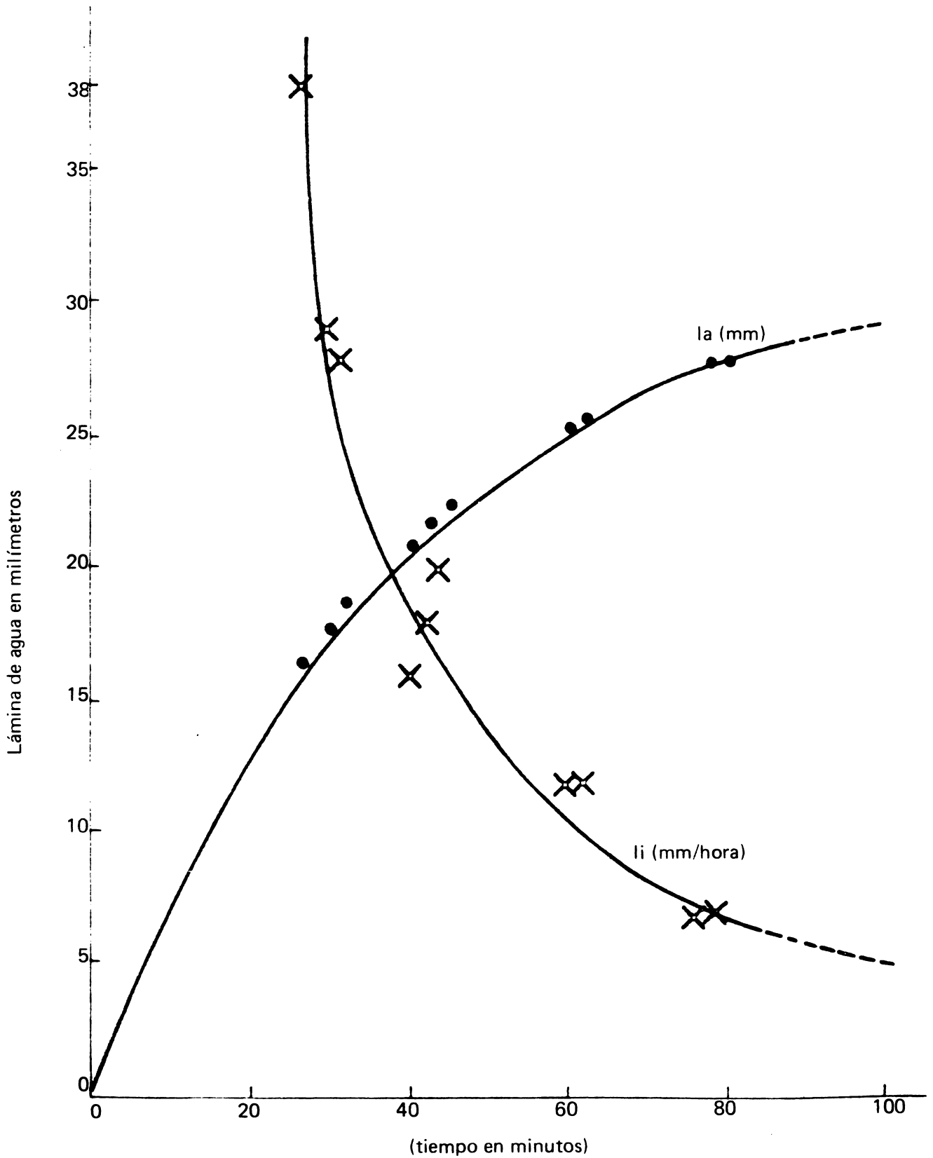
Figura 1. Infiltración instantánea ( li ) y acumulada ( Ia ) en los suelos arenosos de Tacuarembó - Uruguay
