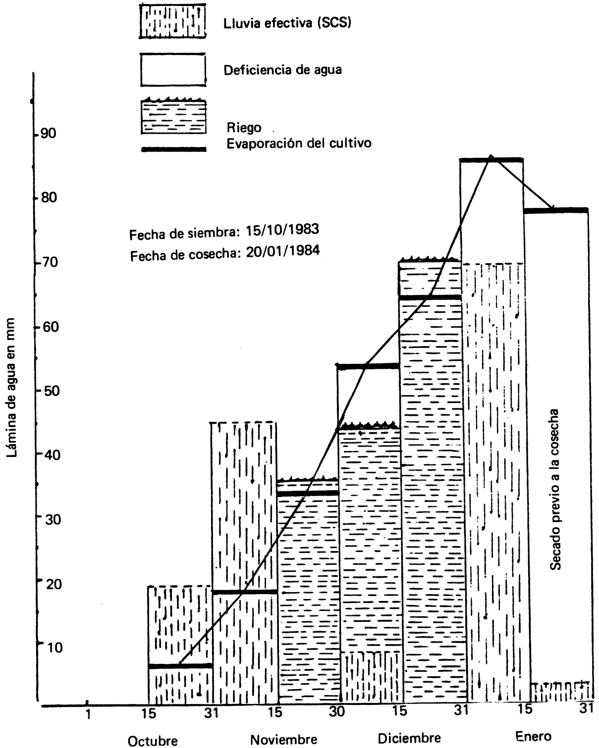
Figura 5. Riego suplementario para papas Kennebeck en Tacuarembó - Uruguay (1983 - 84)
