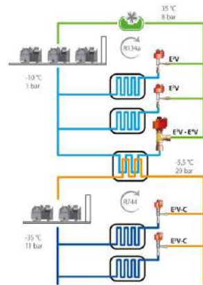
ILUSTRACIÓN 59. SISTEMA DE CO2 SUBCRÍTICO EN CASCA DA.
