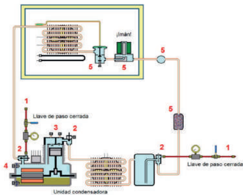
ILUSTRACIÓN 40. PUNTOS SUSCEPTIBLES DE FUGA.
