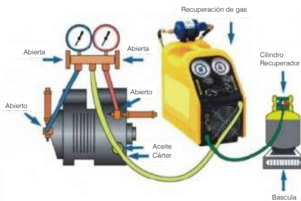
ILUSTRACIÓN 33. MÉTODO DE RECUPERACIÓN EN FASE DE VAPOR.
