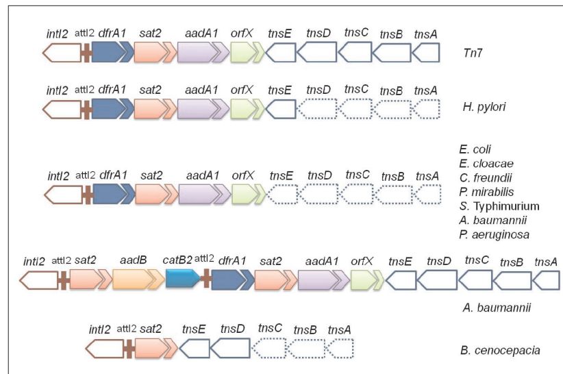
Figura 5. Arreglos en integrones clase 2 descritos en Argentina. Estructura del transposón Tn7 (44, 109) y de distintos arreglos publicados o presentados en Argentina (22, 79, 88-90). Las líneas de puntos en los genes tns implican que no fueron investigados o detectados en todos los casos. En el gráfico se mencionan las especies bacterianas donde fueron descritos.
