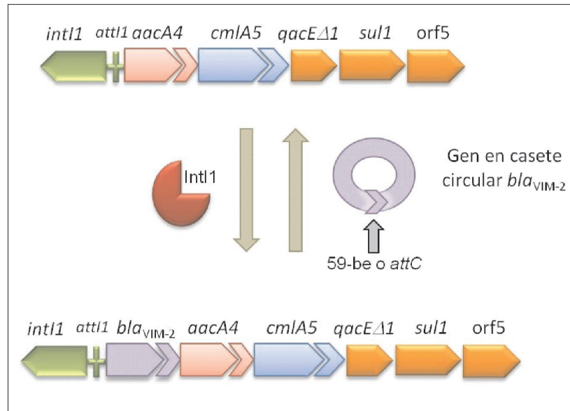
Figura 3. Modelo de integración y escisión de casetes. Proceso por el cual los genes en casete circulares de resistencia a antibióticos se insertan preferencialmente en el sitio específico att1 en un integrón clase 1. Se seleccionó bla VIM-2 (que codifica resistencia a carbapenemes) como ejemplo de gen que se va a incorporar. Dentro de la región variable contamos, además, con genes casete que codifican resistencia a aminoglucósidos ( aacA4 ) y a cloranfenicol ( cmIA5 ). Además, se muestra la estructura del gen en casete circular bla VIM-2 , donde se destaca el sitio de reconocimiento de la integrasa 59-be o attC como parte de su estructura. int11 , gen que codifica la integrasa; Int11: integrasa clase 1. Las flechas de los casetes indican la dirección de la transcripción.
