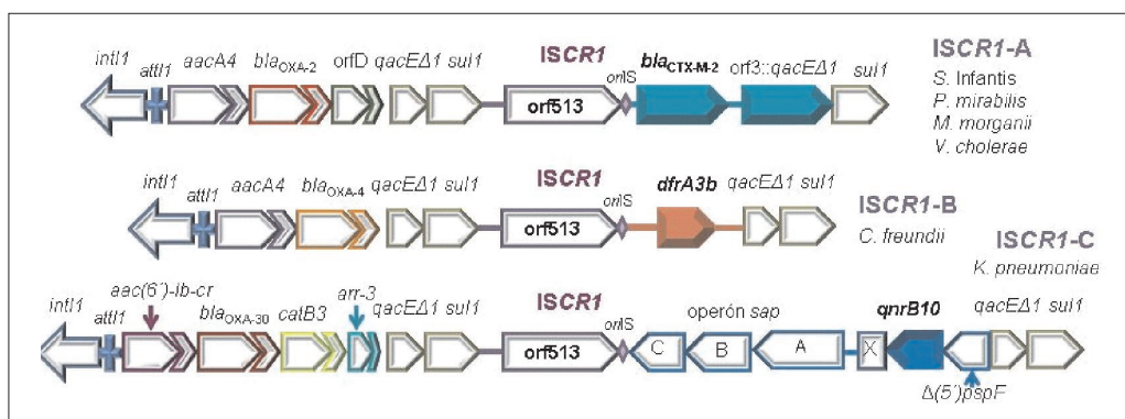
Figura 4. Integrones clase 1 inusuales (complejos): Estructura descrita en Argentina. En cada esquema se destaca en letra violeta el elemento ISCR1 (región conservada de 2,1 kb, incluye el orf513) que se halla estrechamente asociado a estos integrones clase 1 (110, 111). ISCR1-A, -B y -C corresponden a distintos ejemplos de ISCR1 descritos en Argentina, los que se han asociado con alelos que confieren resistencia a cefotaxima (6, 27, 84, 103), a trimetoprima (5) y a ciprofloxacina (85), respectivamente. El integrón esquematizado en ISCR1-C, además del determinante de resistencia a quinolonas asociado qnrB10 , posee el gen en casete aac(6)-Ib-cr , que codifica una nueva variante de la enzima modificadora de aminoglucósidos y que también modifica a la ciprofloxacina, con lo que reduce su actividad. En el gráfico se indican las especies bacterianas donde fueron descritos. Aunque en muchos aislamientos se continuó con la caracterización de la estructura o su entorno, por razones de simplicidad se esquematiza aquí sólo hasta el gen sul1 de la segunda copia del segmento 3'CS.
