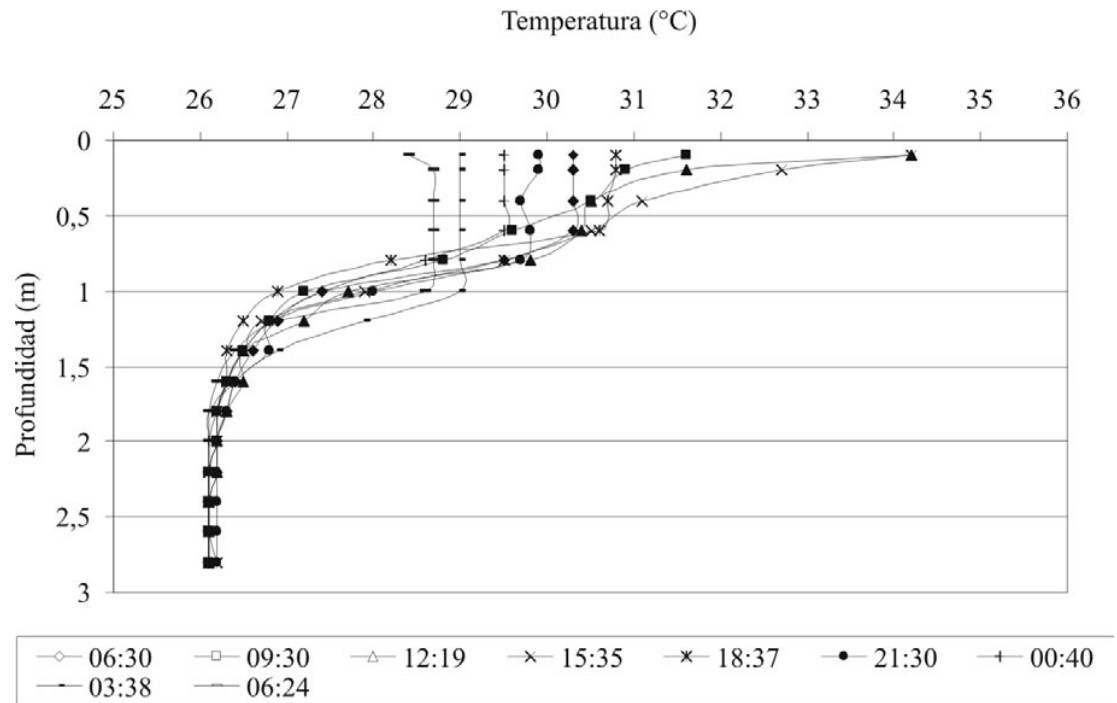
Figura 6 Perfil de temperatura. 12-13 de junio de 2004
