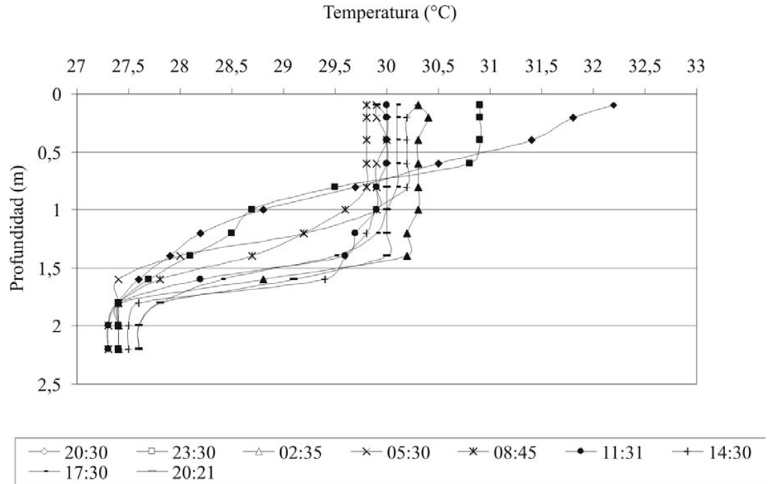
Figura 1 Perfil de temperatura. 19-20 de abril de 2004
