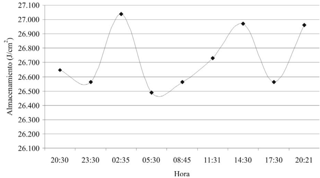
Figura 2 Almacenamiento de calor. 19-20 de abril de 2004
