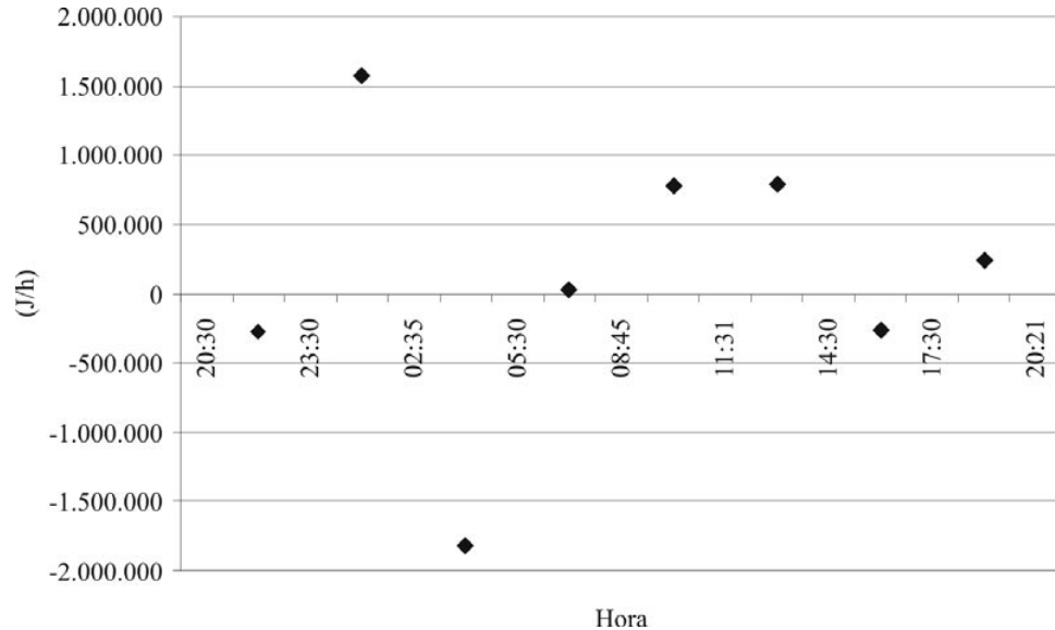
Figura 3 Acumulación de calor. 19-20 de abril de 2004
