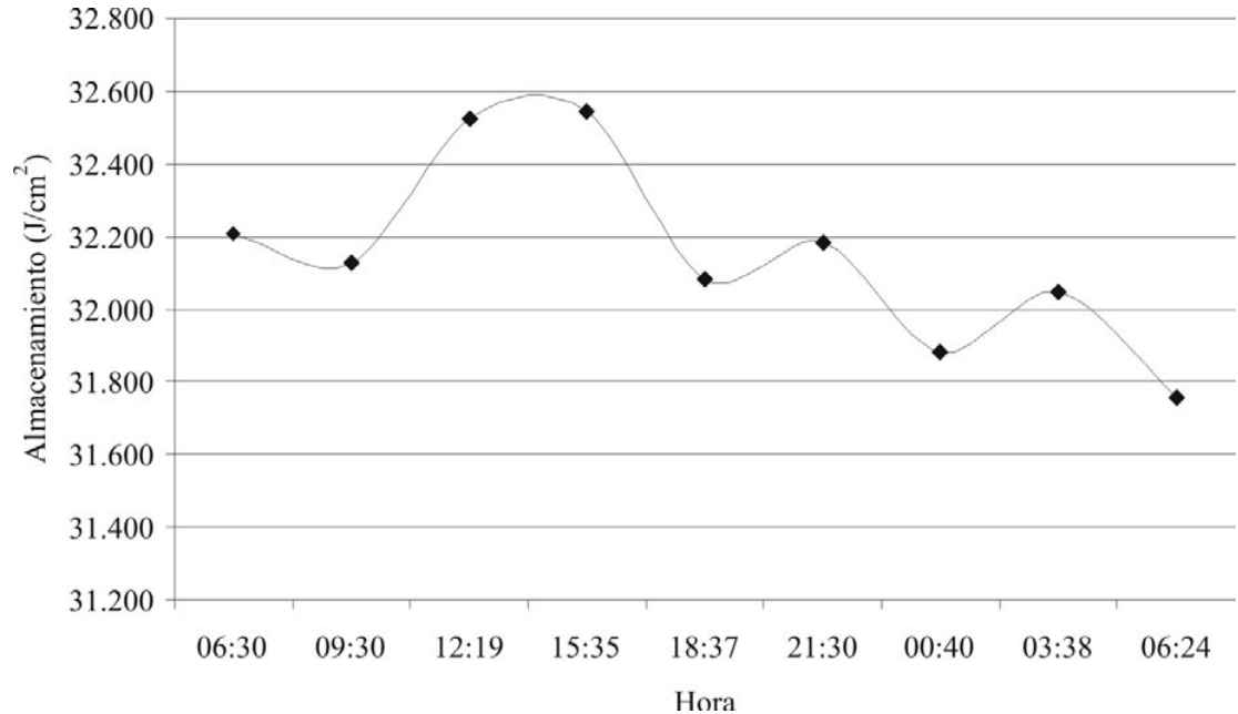
Figura 7 Almacenamiento de calor. 12-13 de junio de 2004
