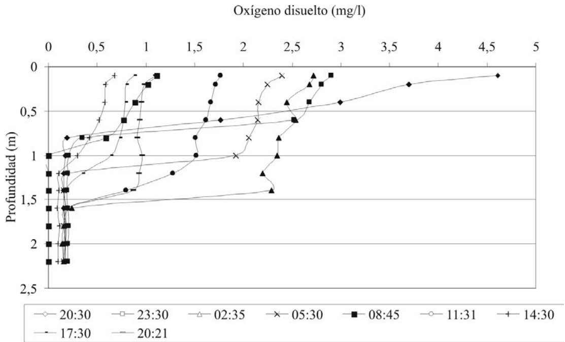
Figura 5 Perfil de Oxígeno. 19-20 de abril de 2004
