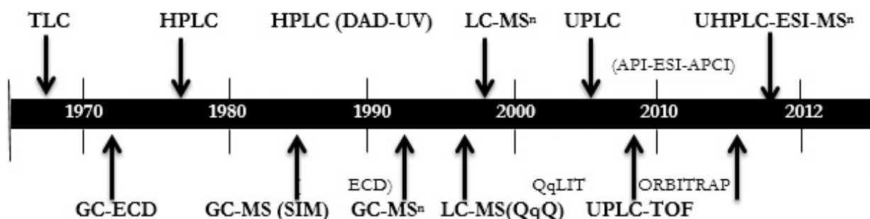
Fig. 1. Evolución de las técnicas analíticas empleadas. QqQ: triple cuadrupolo, QTI: cuadrupolo con trampa de iones, TOF: Tiempo de vuelo, QqTOF: cuadrupolo tiempo de vuelo, TLC: cromatografía en capa fina.
