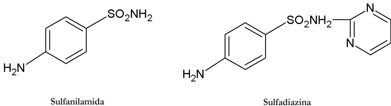
Fig. 2. Estructura Química de las sulfonamidas.
