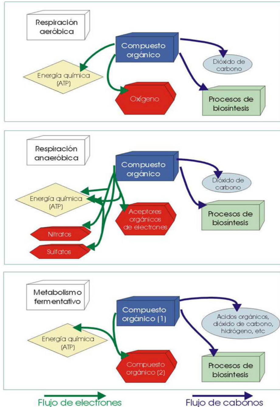
Figura 4. Esquemas de diferentes tipos de metabolismo microbiano
