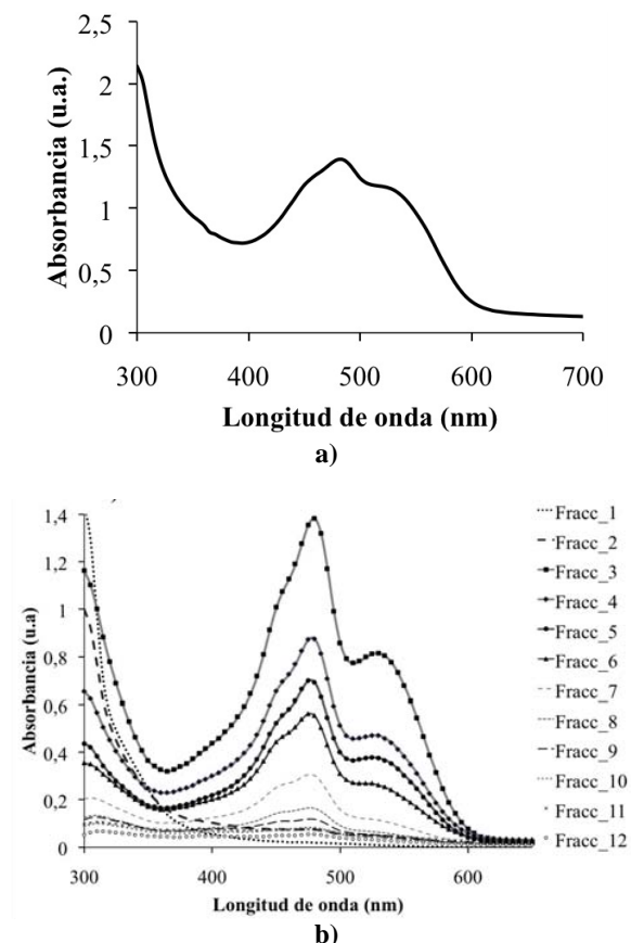
Figura 4. a) Espectro de absorción del barrido de concentraciones del betabel crudo para cuantificar las Betaninas y Betaxantinas. b) Espectros de absorción de las Betacianinas y Betaxantinas obtenidas por CC.
