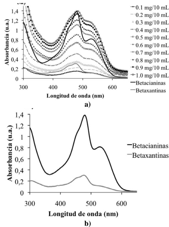
Figura 5. Espectros de absorción de: 1) Crudo de betalainas 1.0 mg/ 10 mL, 2) Espectros de absorción de las fracciones obtenidas por CC.
