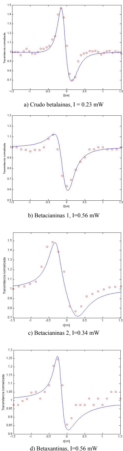
Figura 6. Curvas de barrido en Z para una longitud de onda de 633 nm, para celdas de 20 \mu\text{m} . Las líneas continuas corresponden a las simulaciones numéricas. a) Crudo de las Betalainas, b) y c) Betacianinas, d) Betaxantinas.
