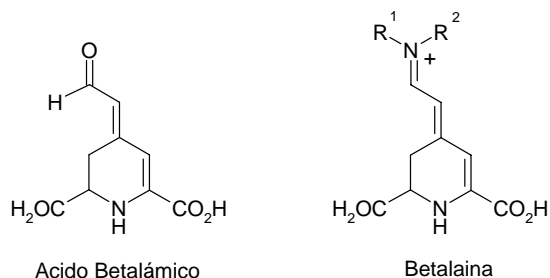
Figura 1. Acido Betalámico y Betalaina.
