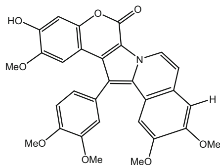
323_lamellarin-η
