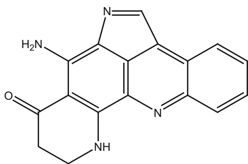
452_Plakinidine
