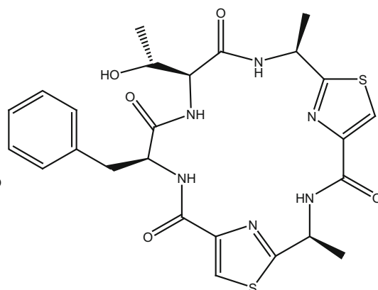
29_Didmolamide B
