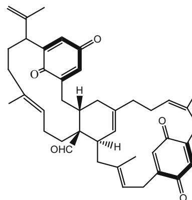
384_longithorone F
