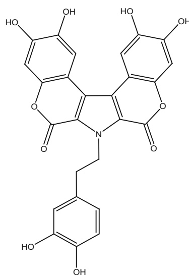
270_ningalin F
