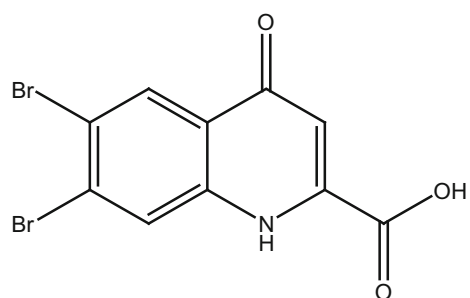
502_Caelestine B
