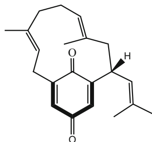
382_longithorone D
