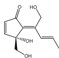
465_cyclopentenones 2
