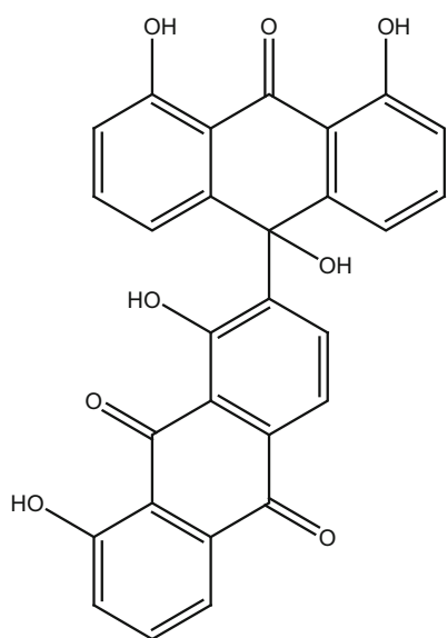
174_albopunctatone
