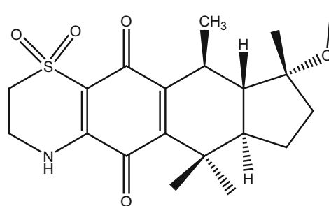
262_conithiaquinones B
