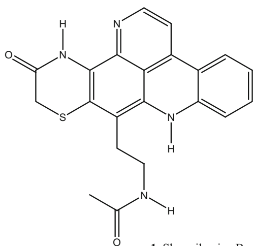
1_Shermilamine B
