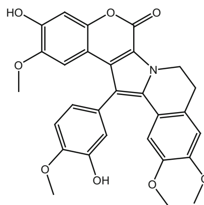
202 _Lamallerin U
