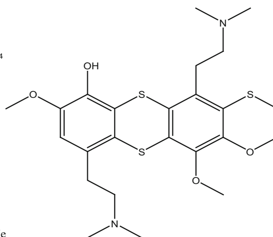
72_Lissoclibadin 6
