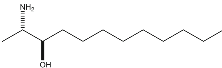
131 _(2S, 3R)-2-Aminododecan-3-ol
