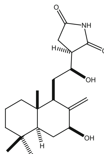
375_haterumaimides Q
