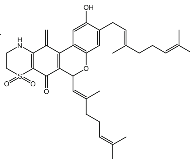
260_thiaplidiaquinones B
