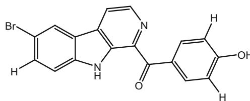
46 Eudistomin Y4
