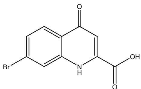
501_Caelestine A
