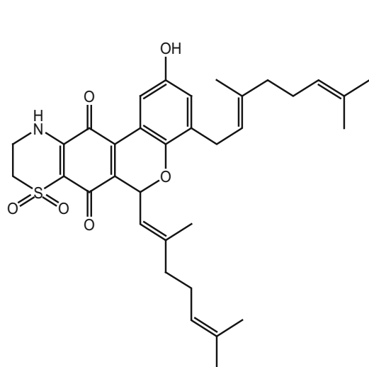
259_thiaplidiaquinones A
