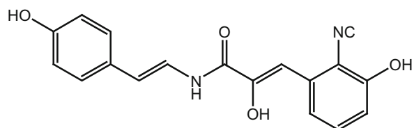
289 _botryllamides H
