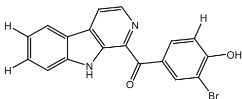
45 Eudistomin Y3
