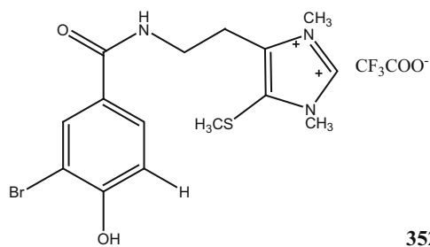
351_leptoclidinamine F
