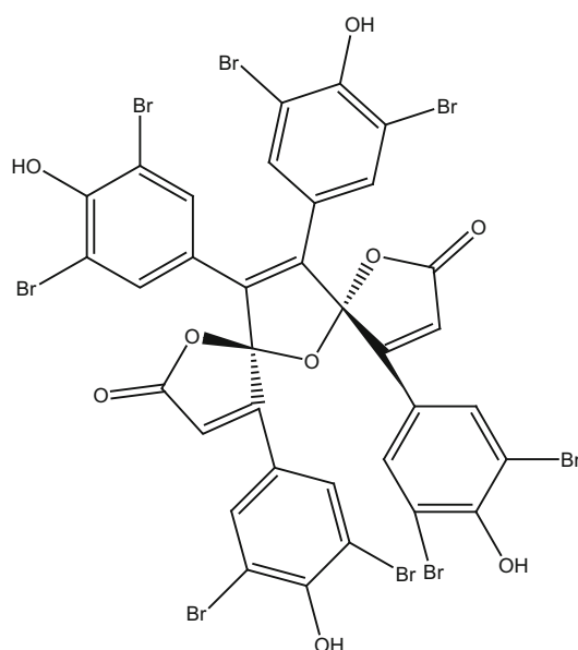
138 prunolide A
