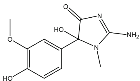
505_Zorrimidazolone
