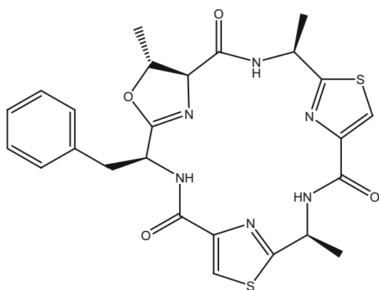
28_Didmolamide A
