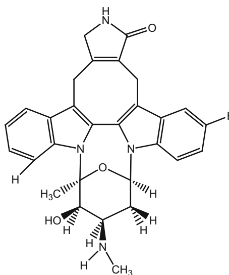
280_3-OH-staurosporine
