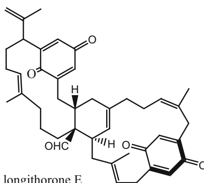
383_longithorone E
