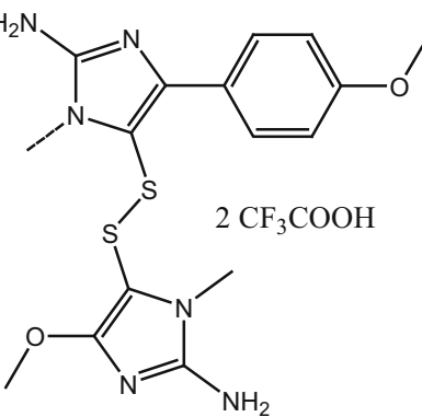
430_polycarpine
