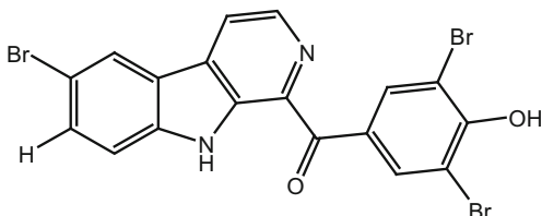
48 Eudistomin Y6
