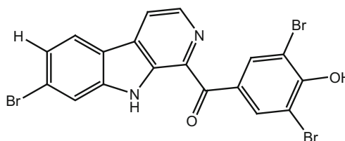
49 Eudistomin Y7
