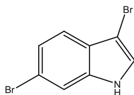
333_3,6-dibromoindole
