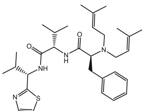
237_virenamides A
