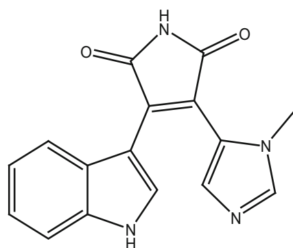
34_didemnimide C
