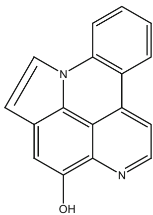
459_arnoamines A
