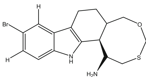
312_eudistomins L
