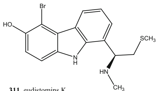
311_eudistomins K
