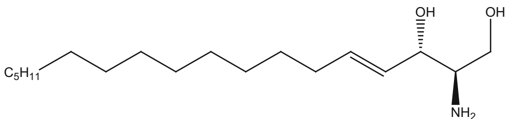
135 _sphingosine
