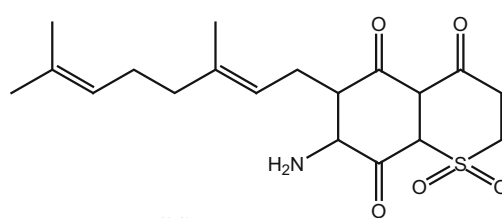
257_aplidinones B
