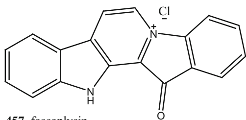
457_fascaplysin
