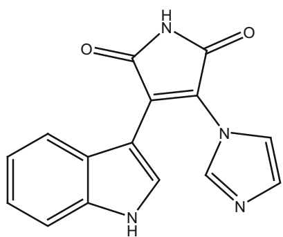
35_isodidemnimide A
