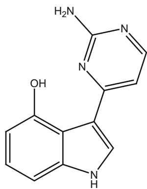
89_Meridianin A
