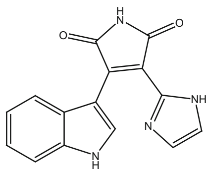
36_neodidemnimide A
