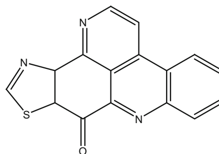
20_kuanoniamines A
