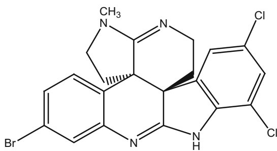
313_perophoramidine
