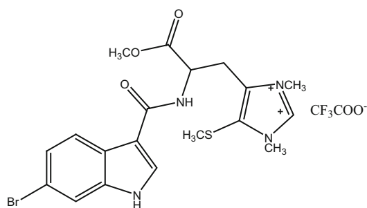
349_leptoclidinamine D
