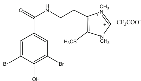
350_leptoclidinamine E
