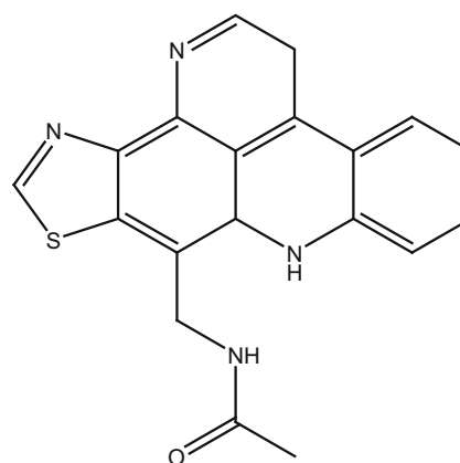
2_Kuanoniamine D
