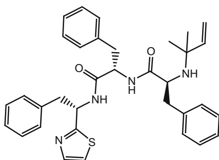
239_virnarnides C
