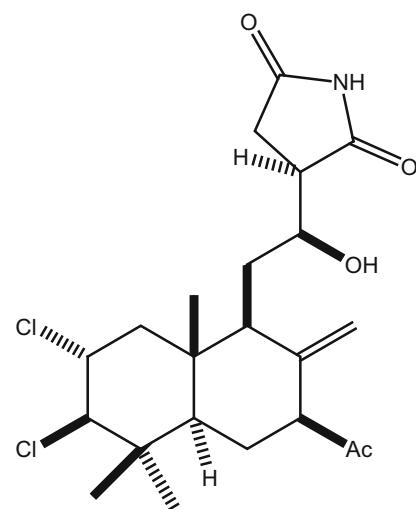
359_haterumaimide A
