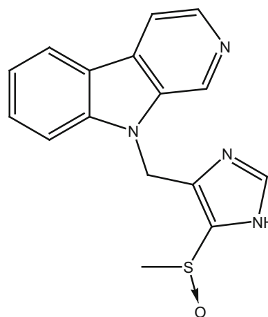
57_Didemnolines D
