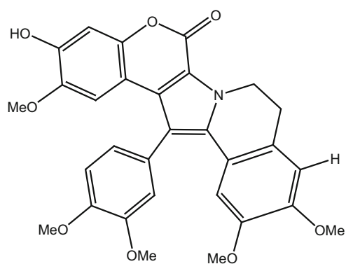
326_lamellarin-J
