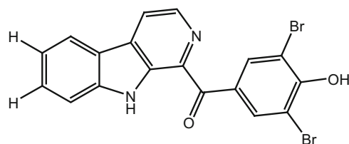
47 Eudistomin Y5
