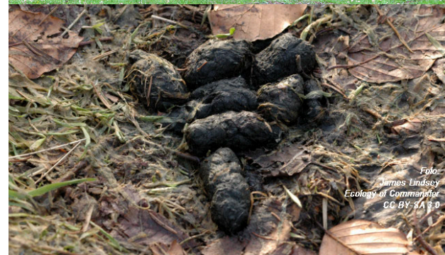
Abb. 2: Fotodokumentation zu Verhaltensweisen des Wildschweins
