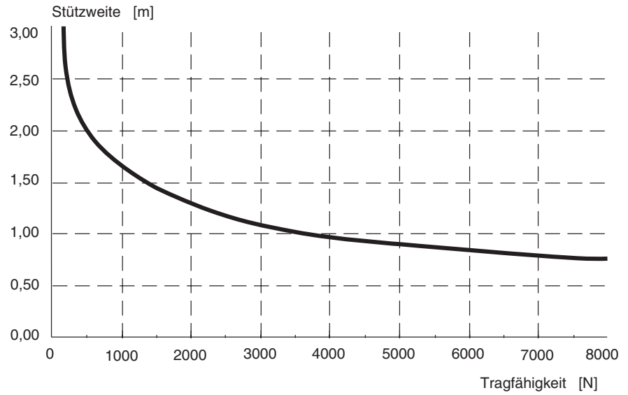
Belastungsdiagramm (Flächenlast Durchbiegung 2 mm)
